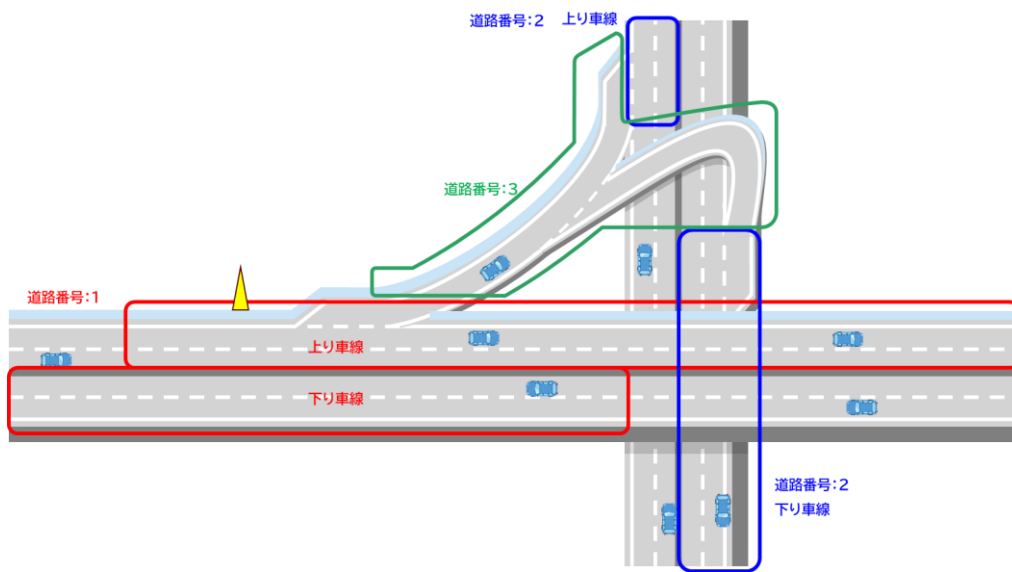
図 A-6 メッセージサイズ試算における想定道路構造
