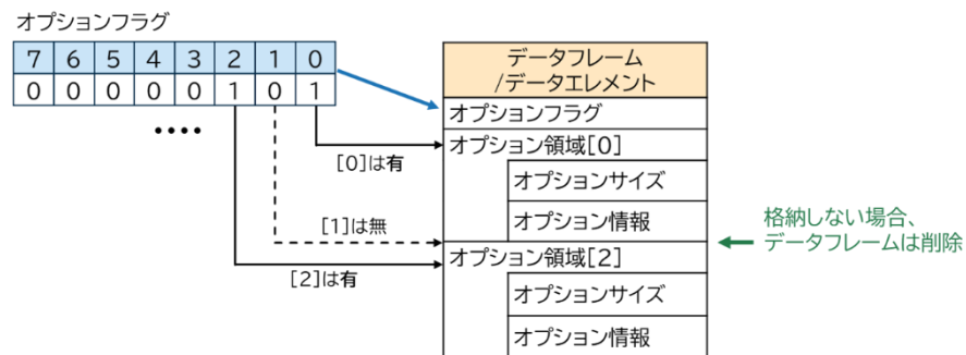
図 A-2 オプション領域の格納例
