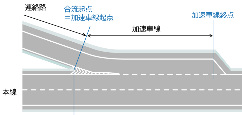
図 A-9 高速道路合流部における合流起点の定義
