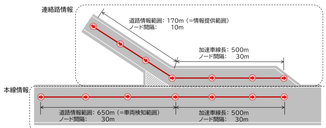
図 A-5 高速道路サービス地点情報の概念図 (合流支援)
