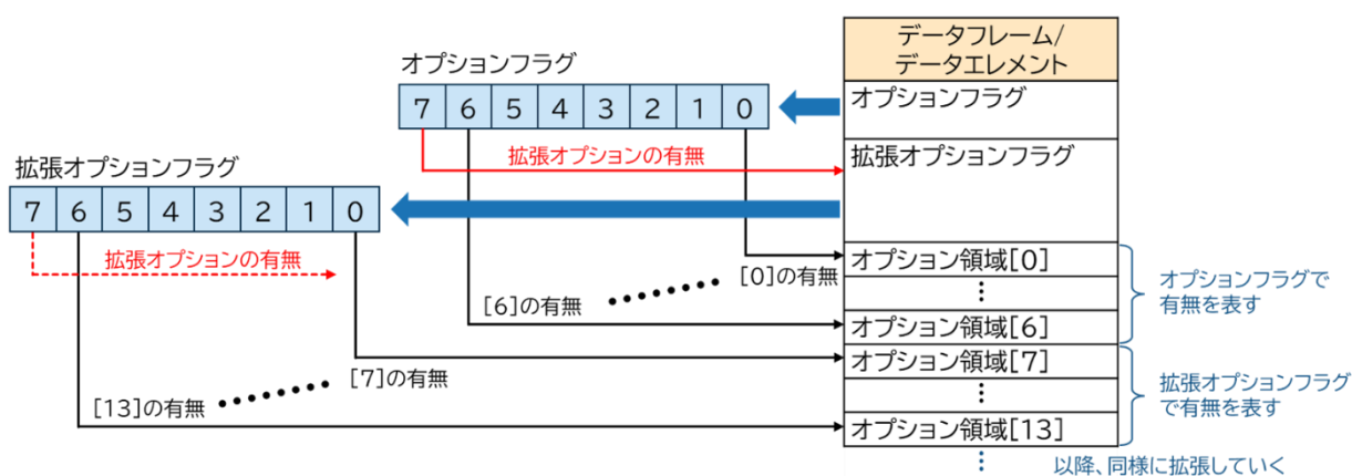
図 A-3 拡張オプション領域
