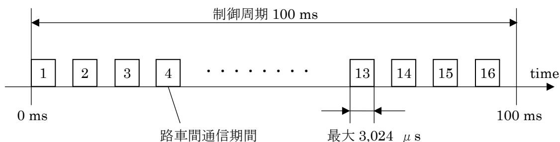
図 A-4 路車間通信期間の配置
