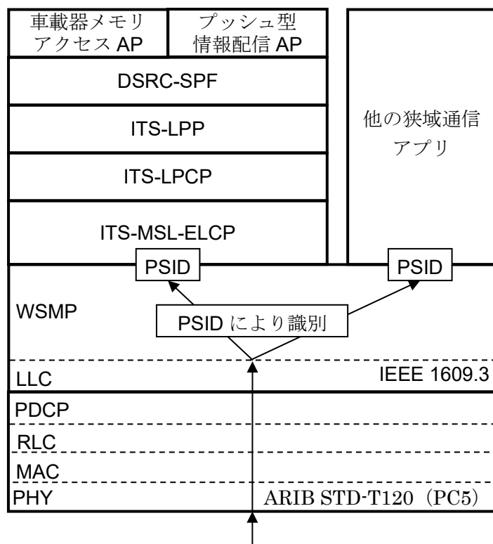
図 2.2-5 ARIB STD-T120 (PC5) における伝送先アプリケーションの識別
