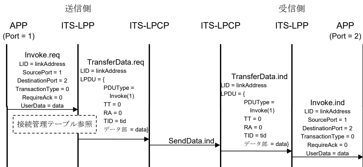
図 3.3-14 データ送信トランザクションサービスの処理シーケンス例
