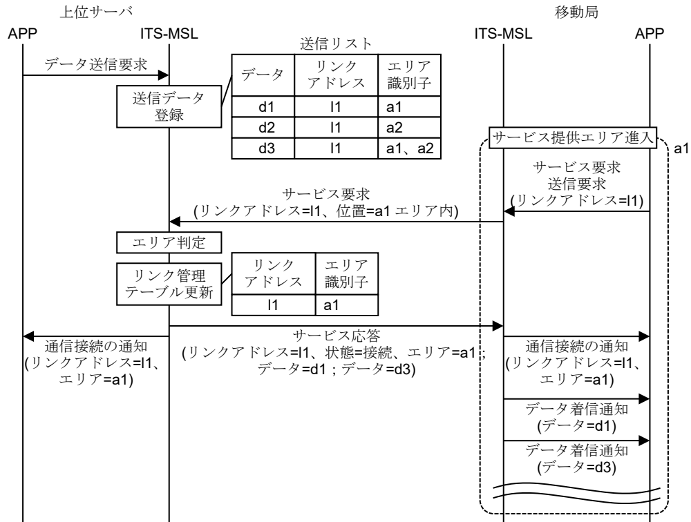
付図 D7-13 転送サービス処理手順の例（サービス提供エリアに進入）
