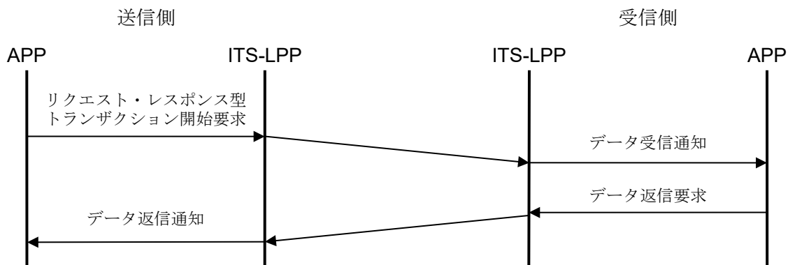
図 3.3-4 リクエスト・レスポンス型トランザクションサービスの例
