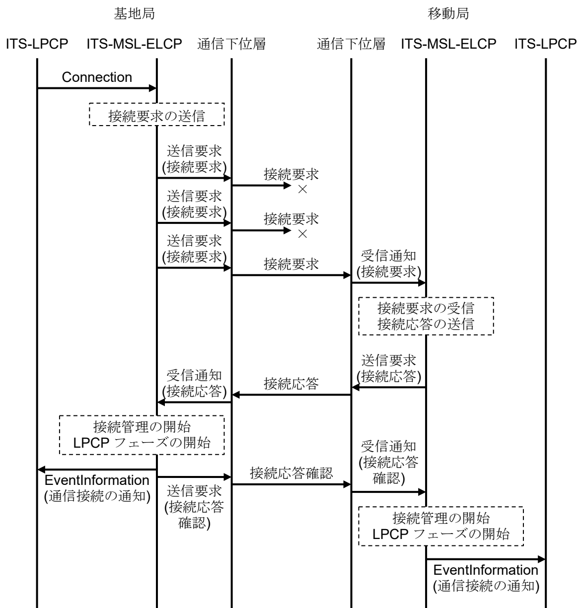
図 3.1-13 通信接続手順の例
