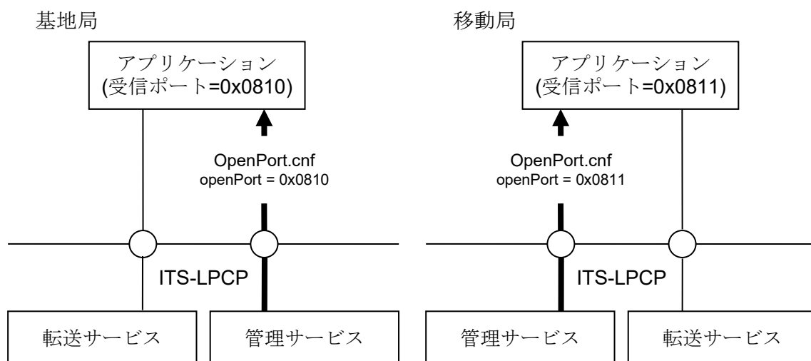
図 3.2-15 アプリケーション登録動作例 (その 2)
