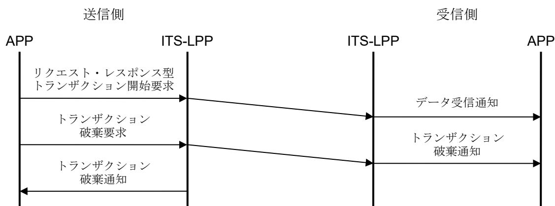
図 3.3-10 トランザクション破棄通知の例
