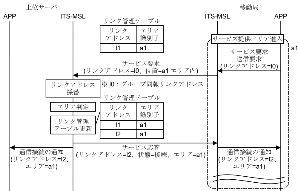
付図 D7-9 通信接続管理手順の例（複数の移動局が同じサービス提供エリアに進入）
