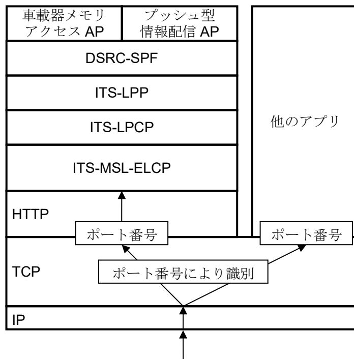
図 2.2-3 ARIB STD-T104・ARIB STD-T120 (Uu) における伝送先アプリケーションの識別
