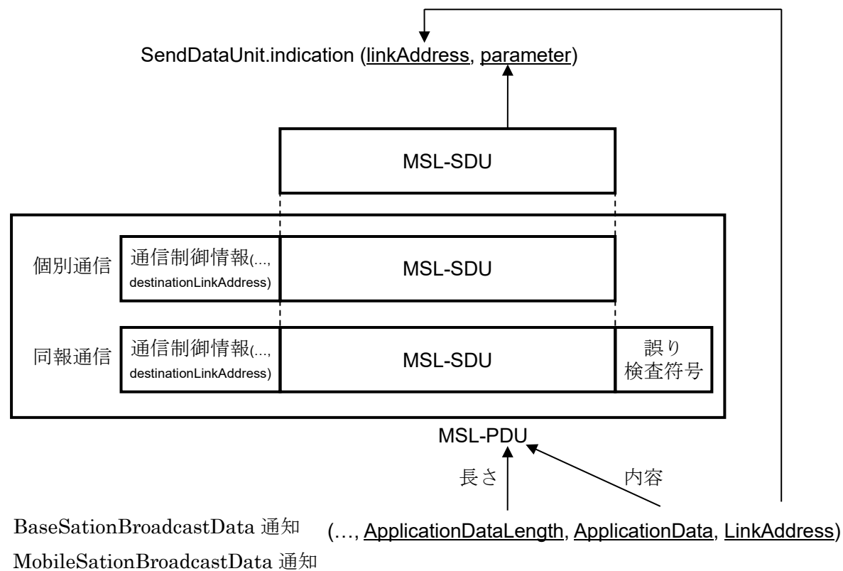
付図 F-2 SendDataUnit.indication における下位層プリミティブへのマッピング
