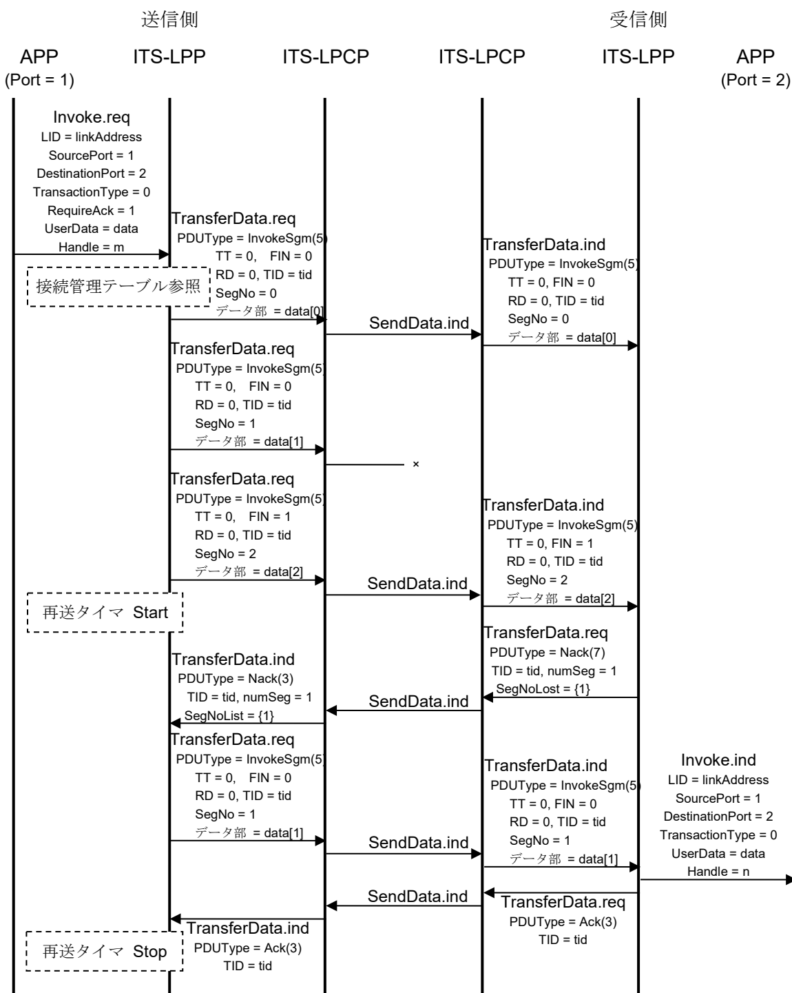
図 3.3-21 分割・組立処理が有効な場合のシーケンス例 (選択的再送処理)
