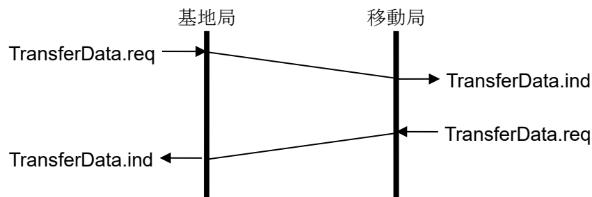
図 3.2-1 データ転送プリミティブの論理関係
