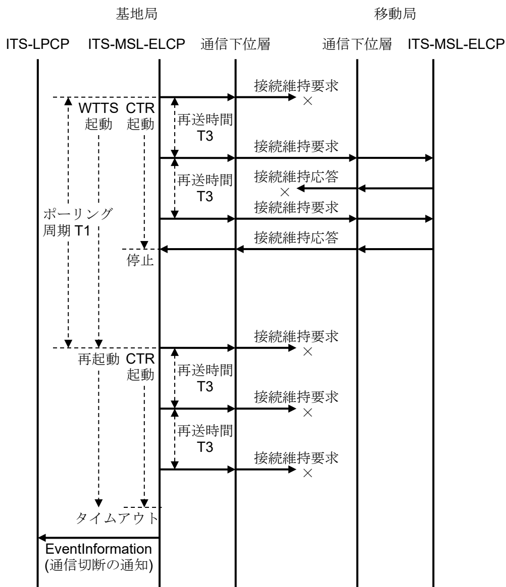
図 3.1-15 接続維持要求の再送制御手順の例
