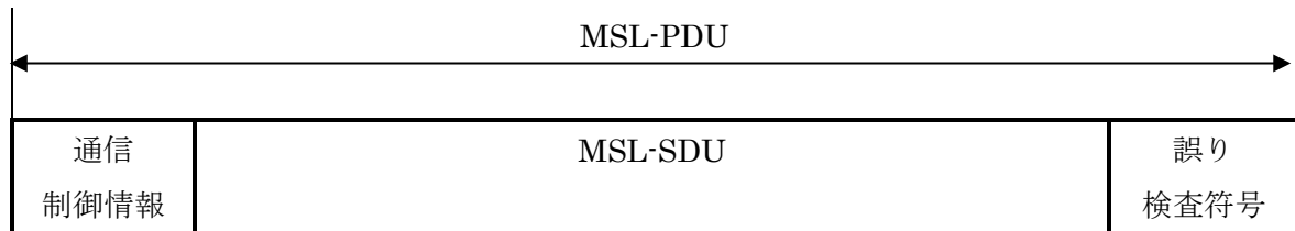
(b) 同報通信の PDU 形式
