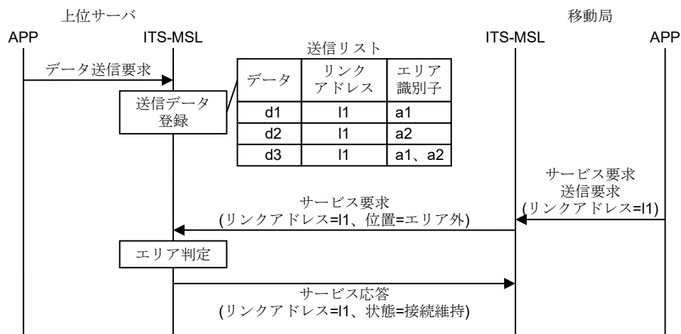
付図 D7-10 転送サービス処理手順の例 (サービス提供エリア外を走行)
