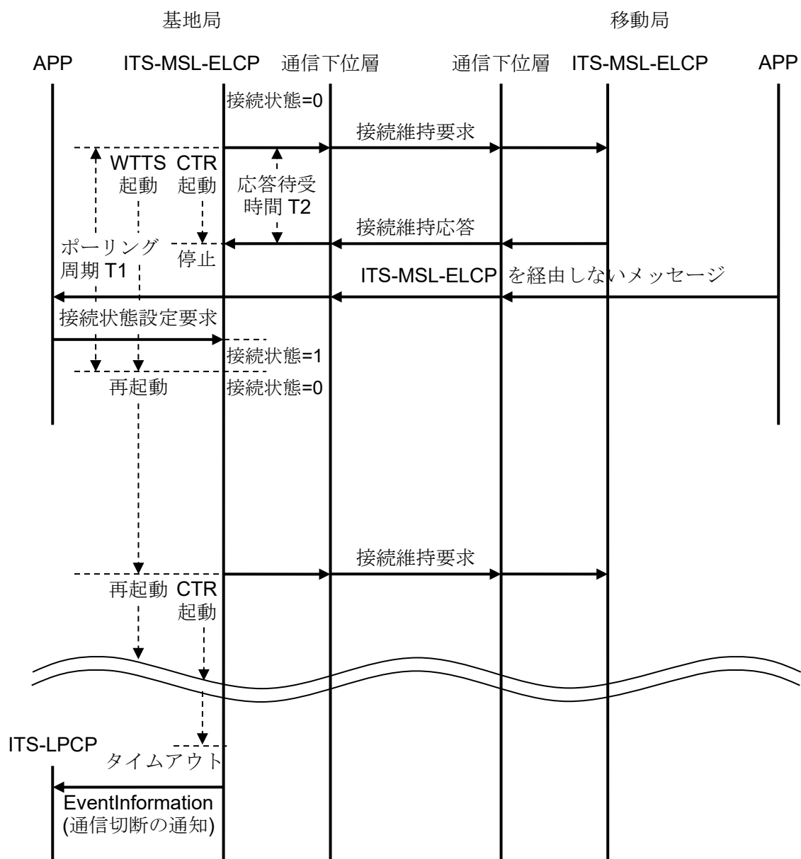
図 3.1 アプリケーションから接続状態を設定する通信接続管理手順の例
