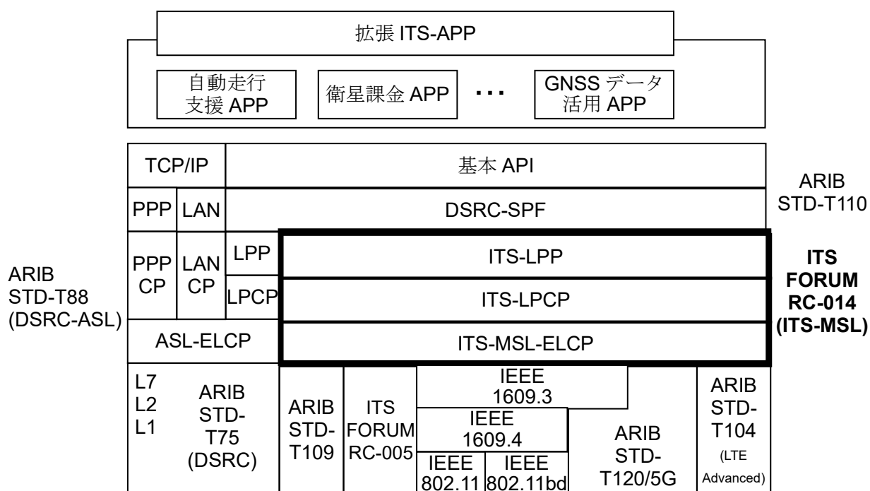
図 1.2-1 ITS プラットフォーム（拡張）のプロトコル構成
