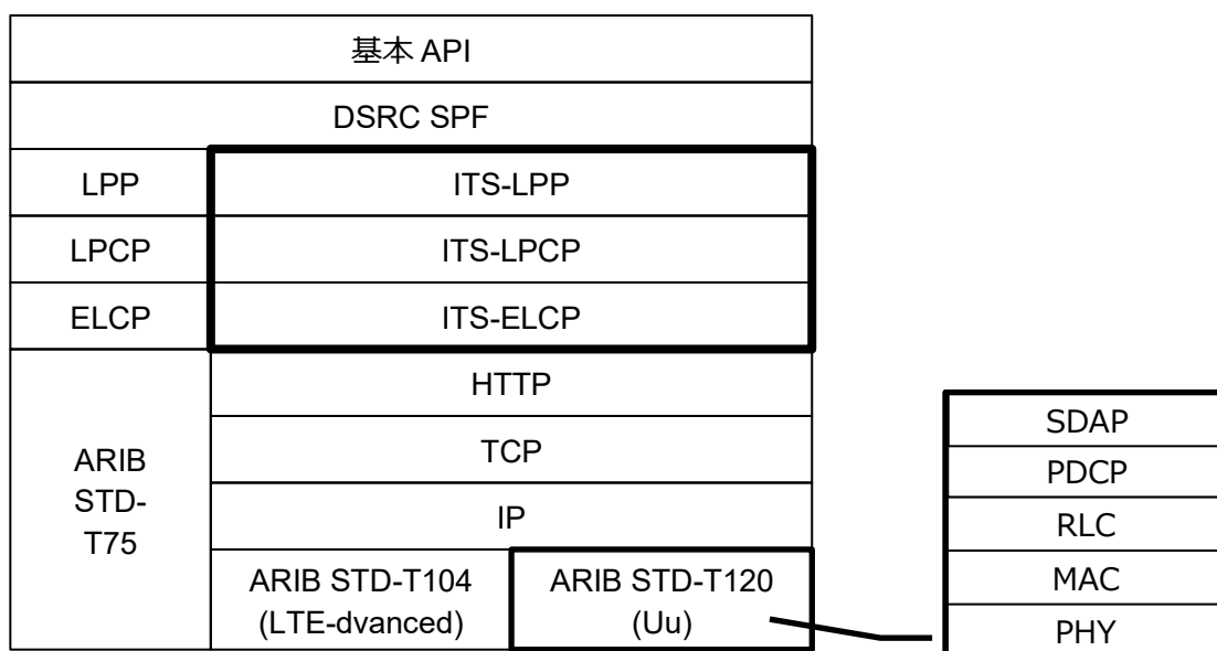
付図 E-2 ARIB STD-T120 (Uu) 適用時のプロトコル構成
