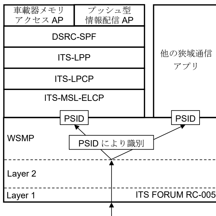
図 2.2-1 ITS FORUM RC-005 における伝送先アプリケーションの識別
