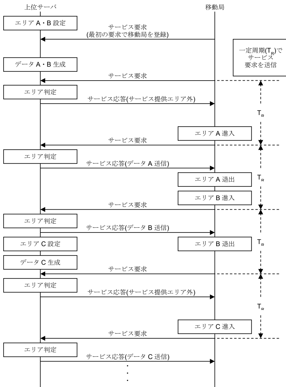
付図 D5-1 上位サーバからデータ配信する処理手順の例 (エリア判定を上位サーバで実施)
