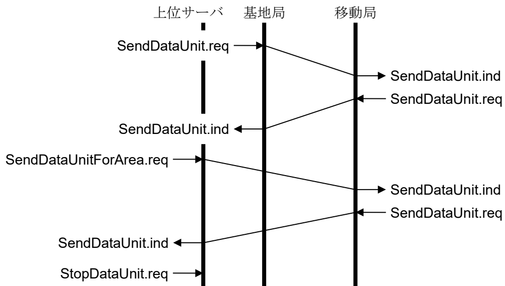
図 3.1-3 通信サービスプリミティブの論理関係
