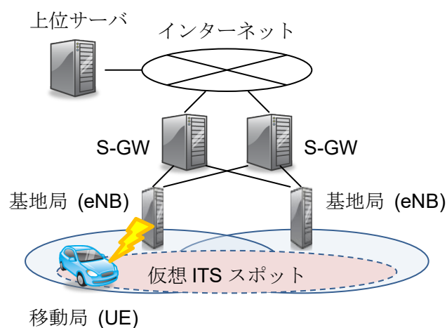
付図 D1-1 LTE-Advanced を使った ITS-MSL の適用イメージ
