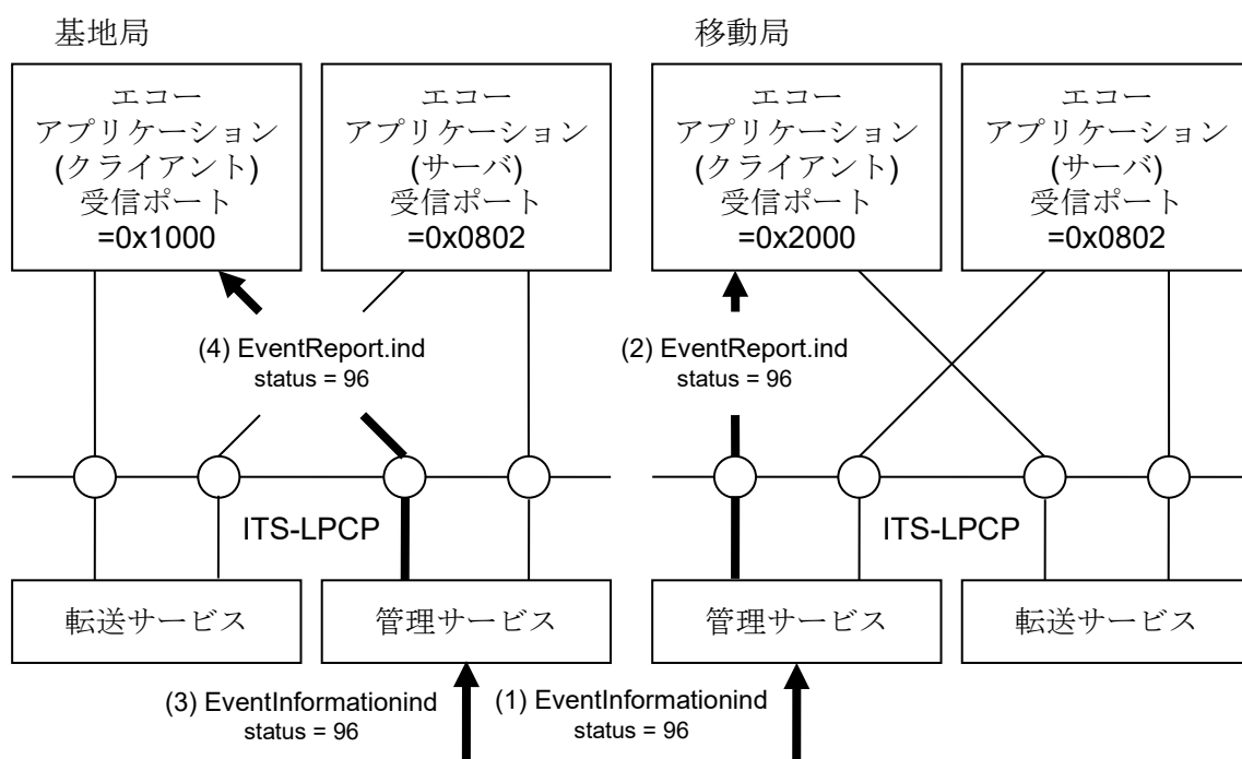
図 3.2-10 初期接続動作 (接続通知)
