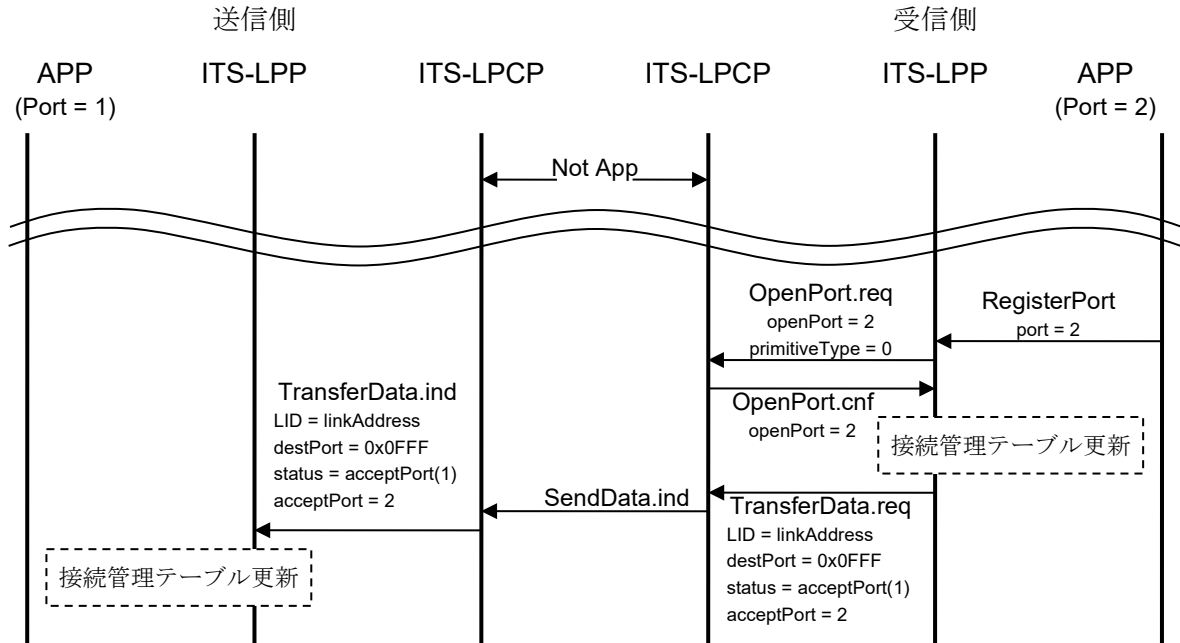
図 3.3-26 受信可能ポート追加手順の例
