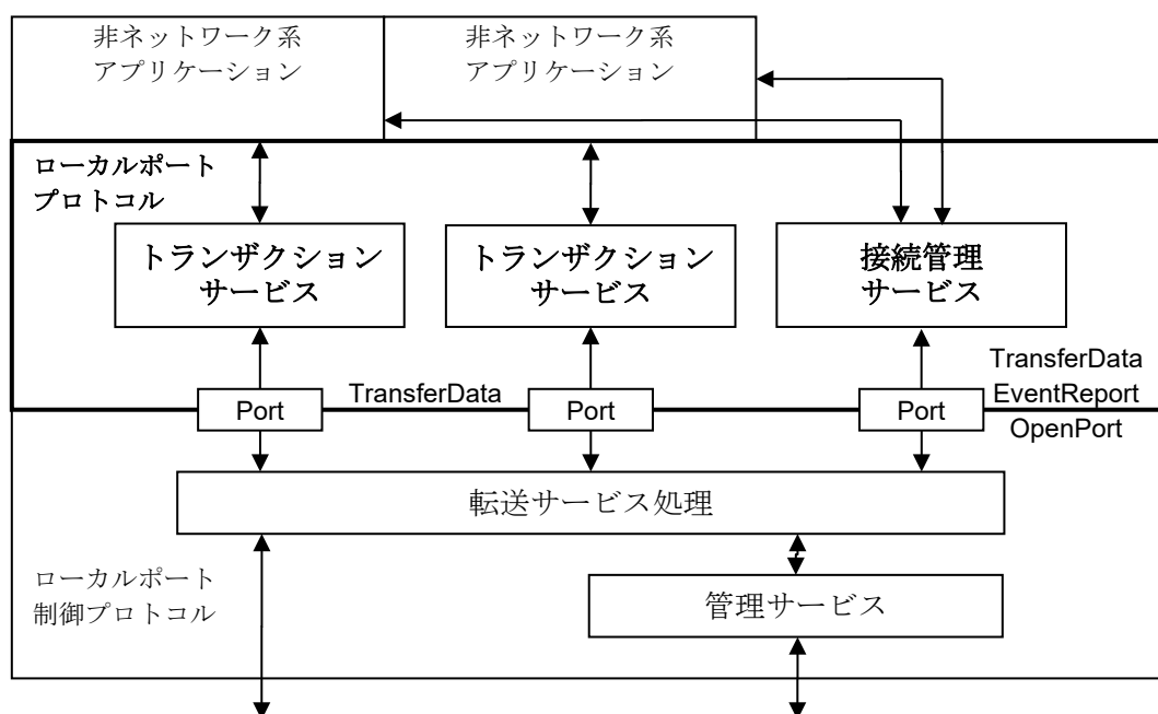
図 3.3-1 LPP の概念図
