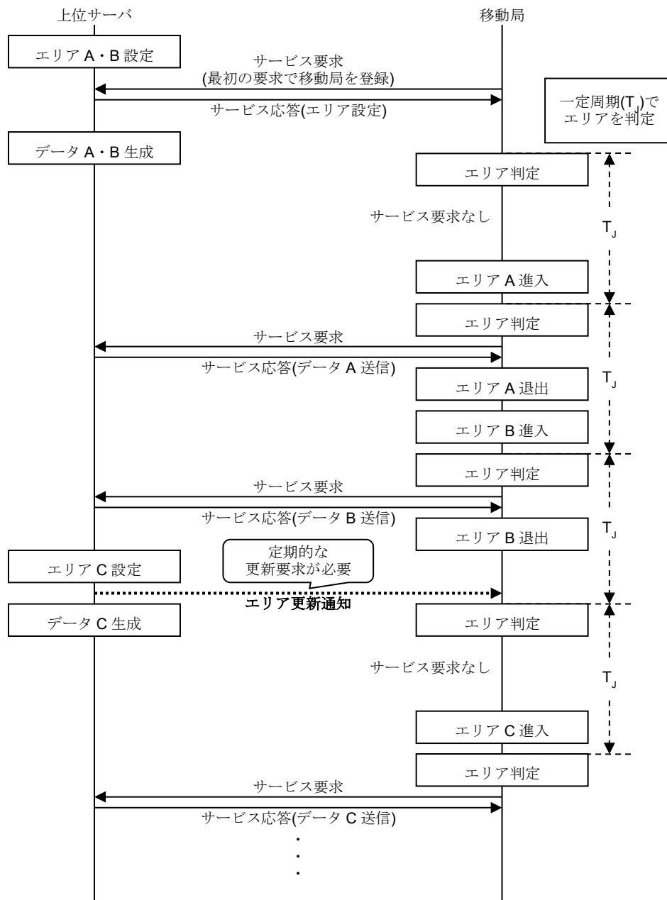
付図 D5-2 上位サーバからデータ配信する処理手順の例 (エリア判定を移動局で実施)
