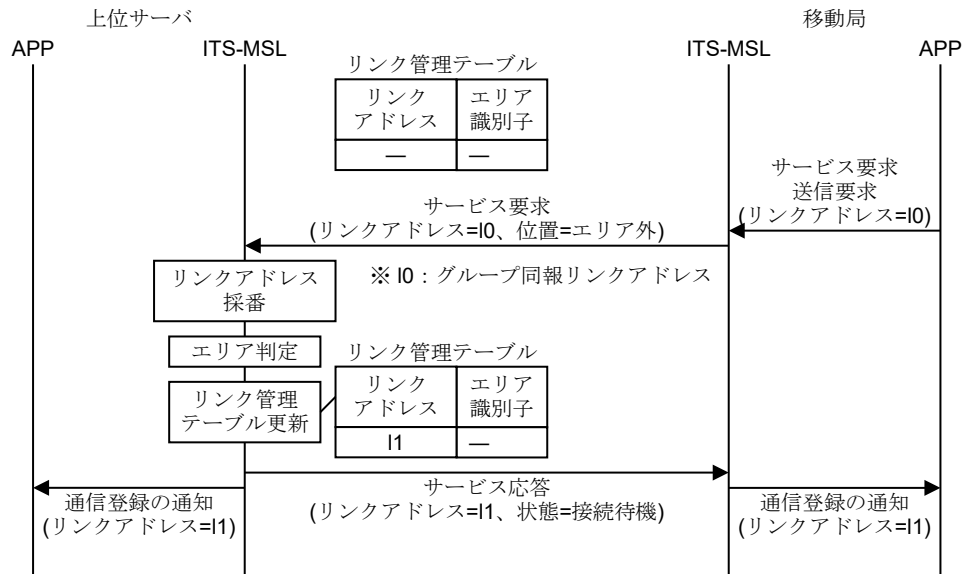
付図 D7-3 通信接続管理手順の例 (サービス提供エリア外でサービス要求開始)
