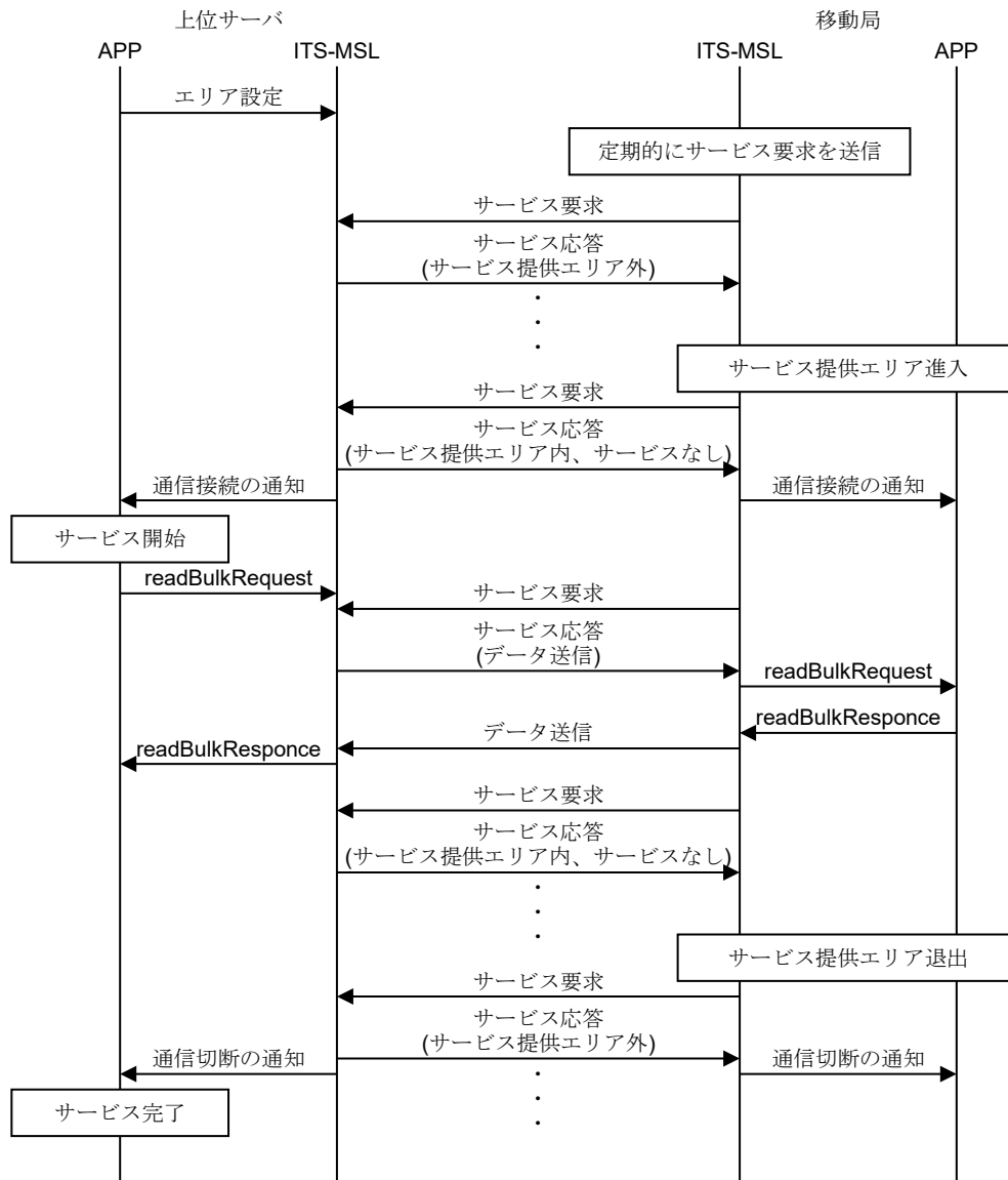
付図 D6-1 ARIB STD-T104 を使った場合の車載器メモリー一括取得の処理手順の例
