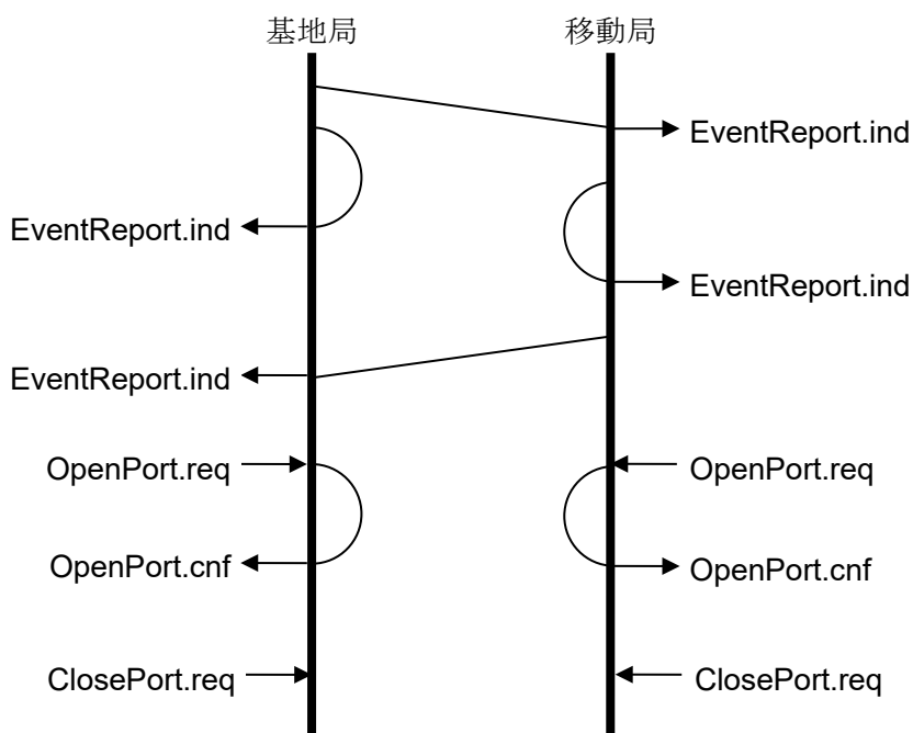
図 3.2-2 管理サービスプリミティブの論理関係
