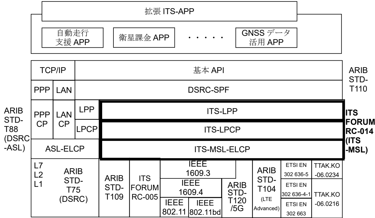
付図 A2-1 ITS プラットフォーム (拡張) のプロトコル構成
