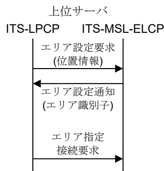
図 3.1-16 エリア設定手順の例
