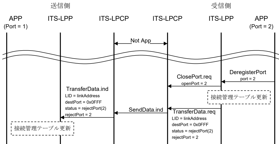
図 3.3-27 受信可能ポート削除手順の例
