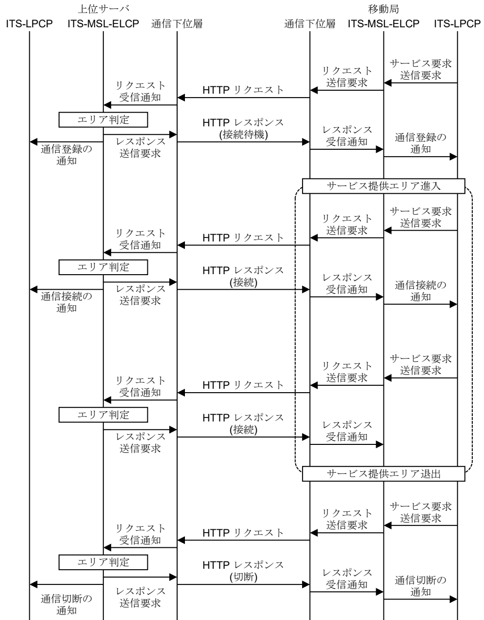
図 3.1-17 通信接続手順の例
