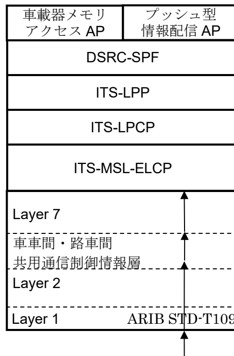
図 2.2-6 ARIB STD-T109 における伝送先アプリケーションの識別
