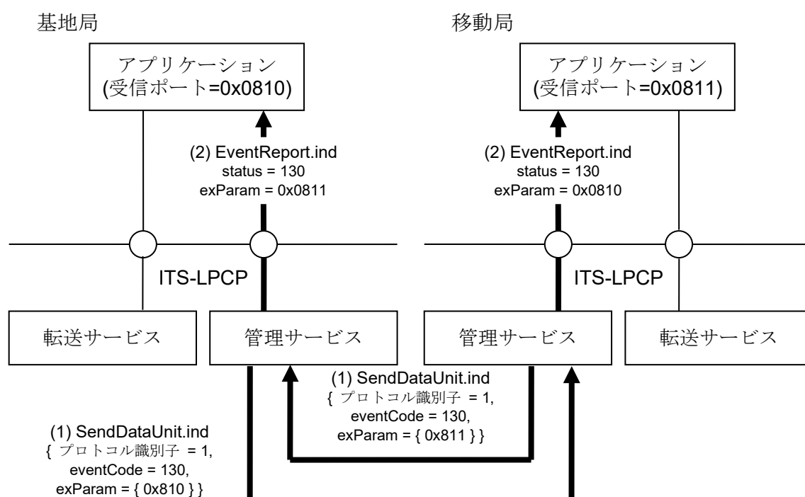
図 3.2-17 初期接続動作 (受信可能ポートリスト交換)
