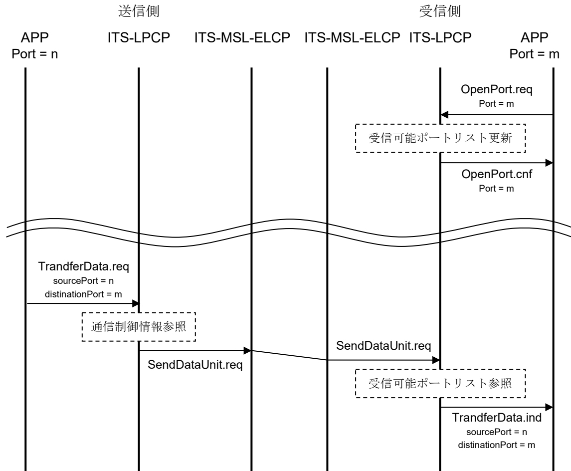
図 3.2-5 データ転送処理手順の概略
