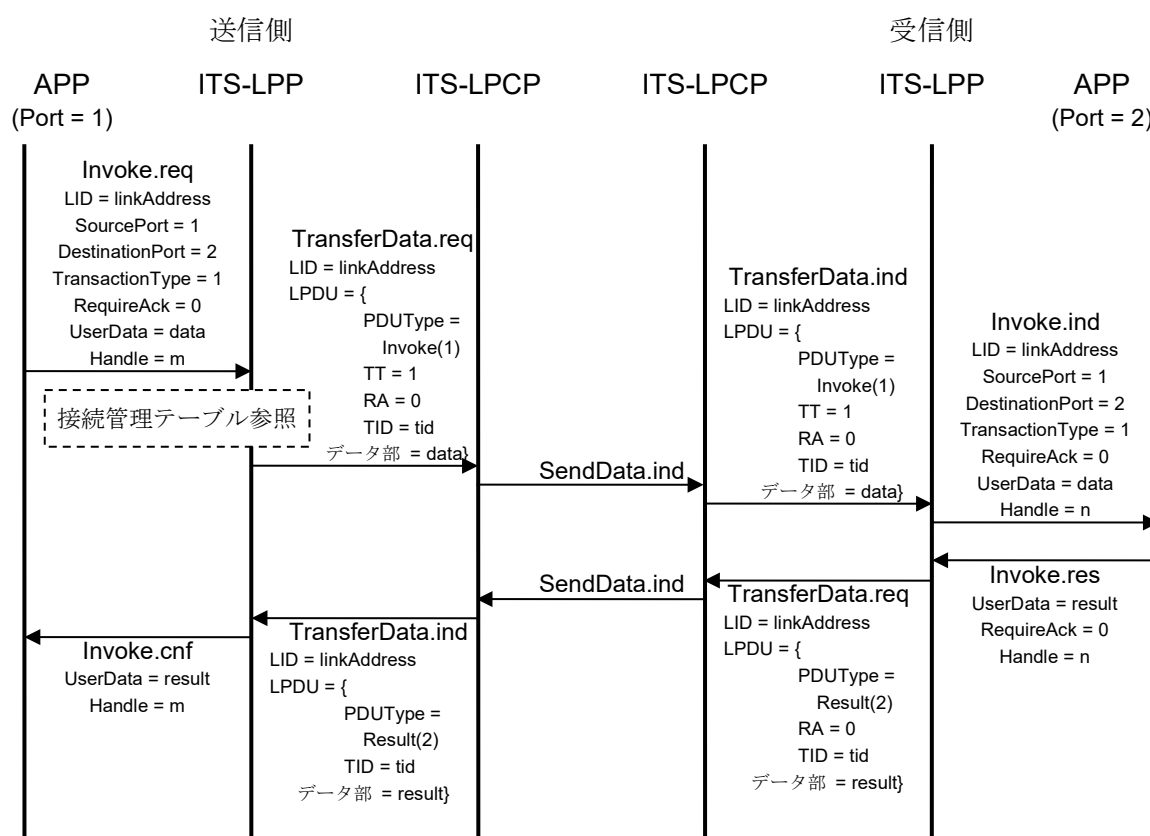
図 3.3-15 リクエスト・レスポンス型トランザクションサービスの基本処理シーケンス例
