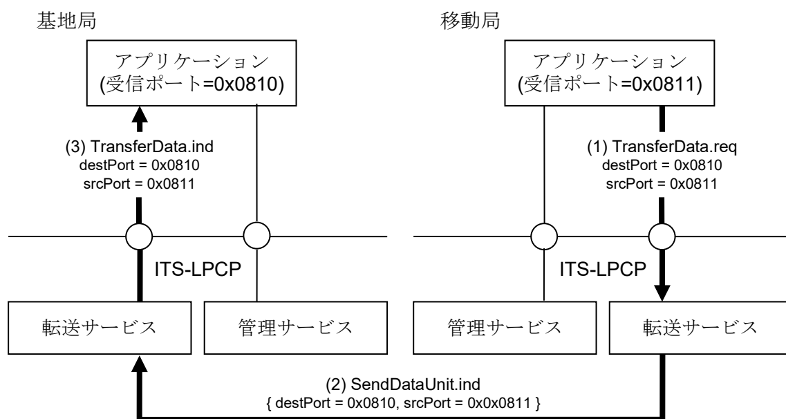
図 3.2-19 データ転送動作例 (移動局→基地局)
