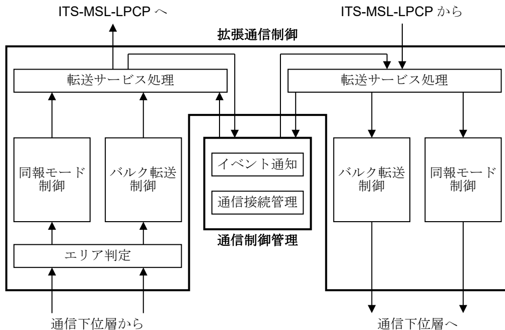
図 3.1-1 上位サーバにおける ITS-MSL-ELCP のエンティティ構成
