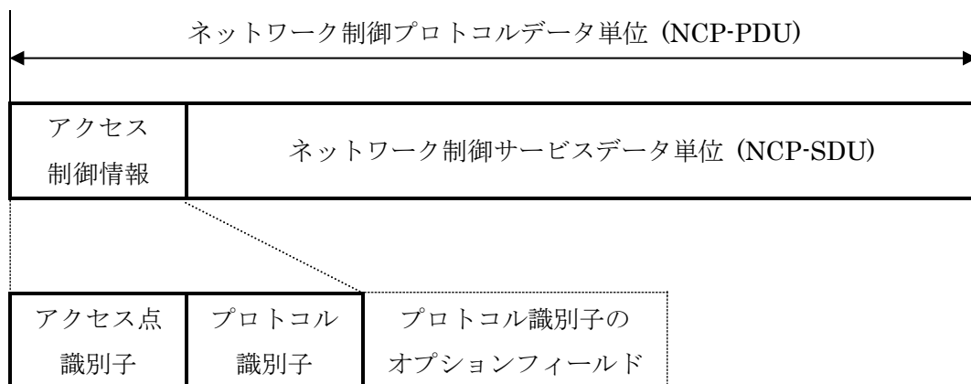
図 3.1-12 通信制御管理の PDU の構成
