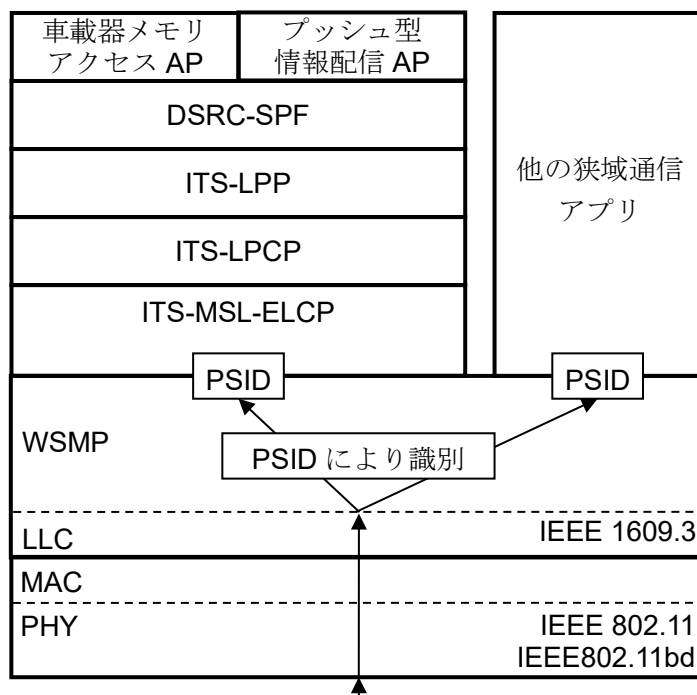
付図 C1-1 IEEE802.11・IEEE 802.11bd におけるコネクションの識別
