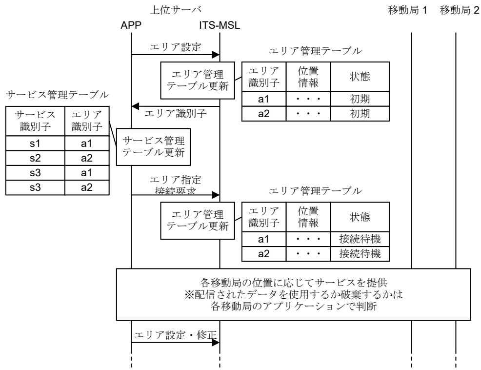
付図 D7-2 サービスとサービス提供エリアの管理手順の例
