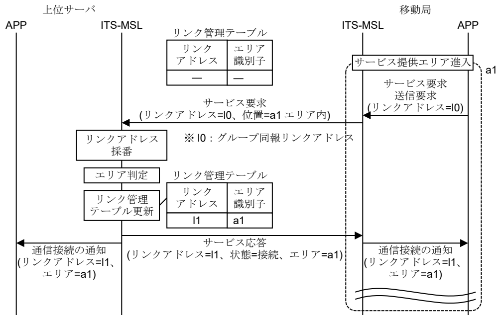
付図 D7-4 通信接続管理手順の例 (サービス提供エリア内でサービス要求開始)
