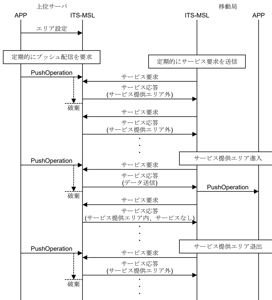
付図 D6-2 ARIB STD-T104 を使った場合のダウンリンク常時同報通信の処理手順の例
