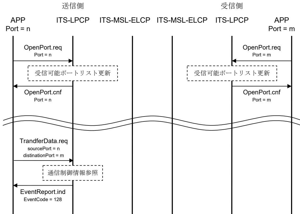
図 3.2-6 通信が接続されていない場合の処理手順の概略
