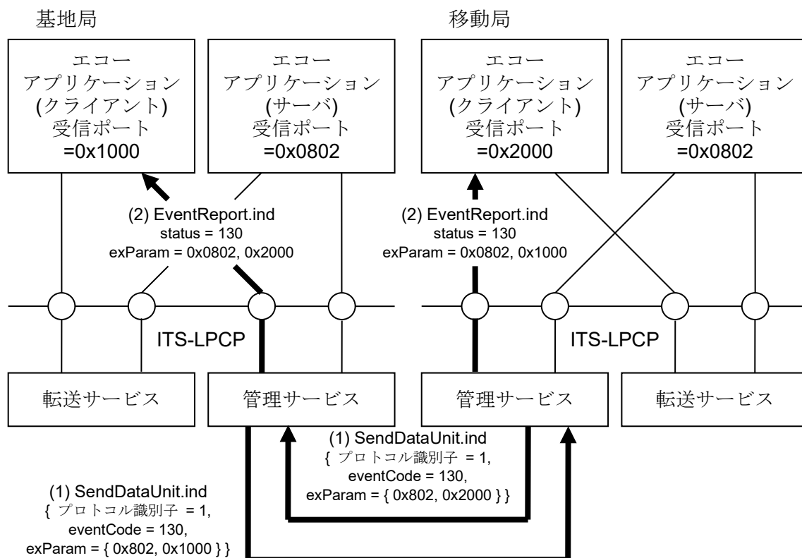
図 3.2-11 初期接続動作 (受信可能ポートリスト交換)
