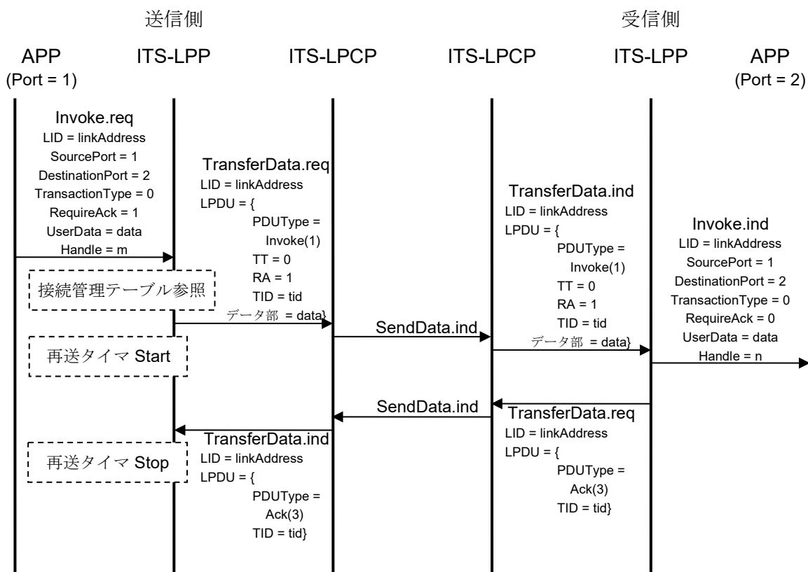
図 3.3-17 再送処理が有効な場合のデータ転送手順（基本シーケンス）
