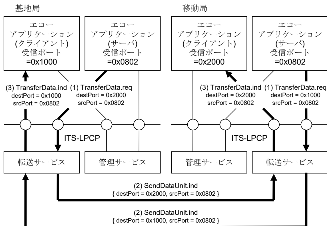
図 3.2-13 データ転送動作例 (エコー応答)
