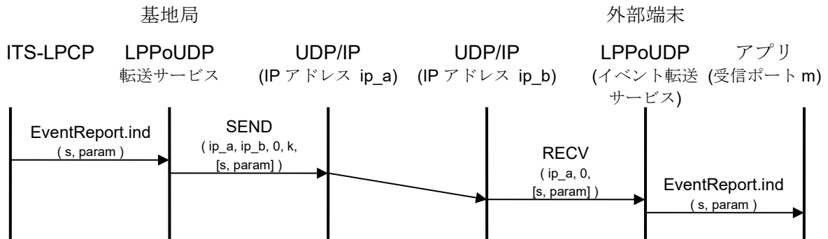
図 3.3-36 EventReport.ind シーケンス
