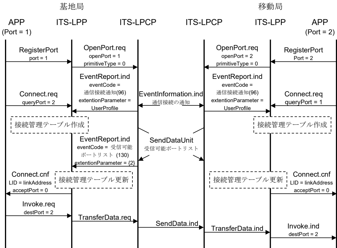
図 3.3-12 ITS-LPP の初期接続手順
