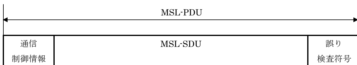
(b) 同報通信の PDU 形式
