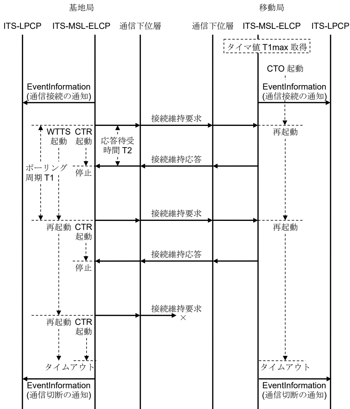
図 3.1-14 通信接続管理手順の例
