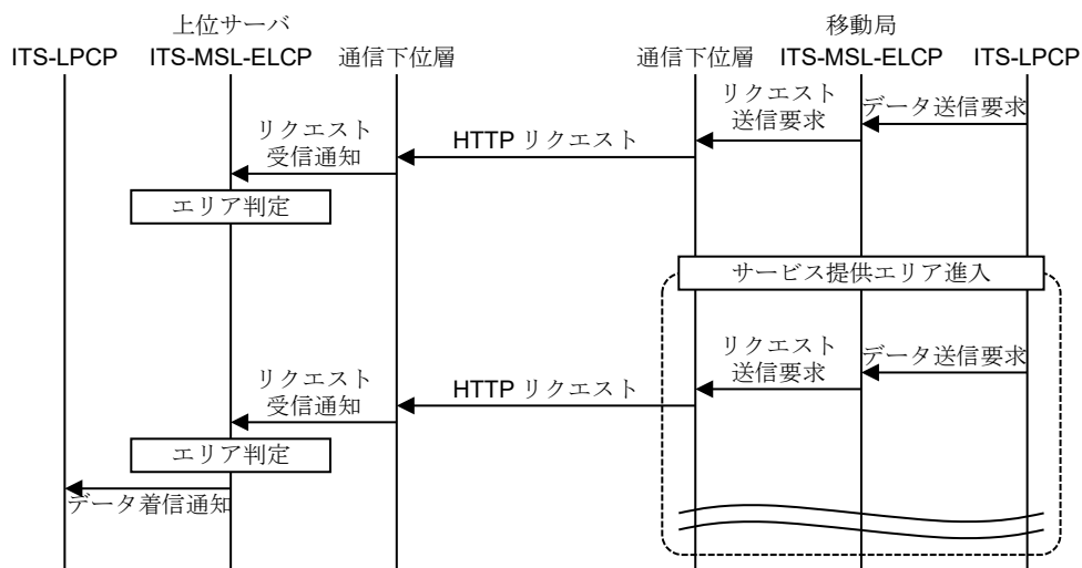
図 3.1-9 移動局から上位サーバへの転送サービス処理手順の例
