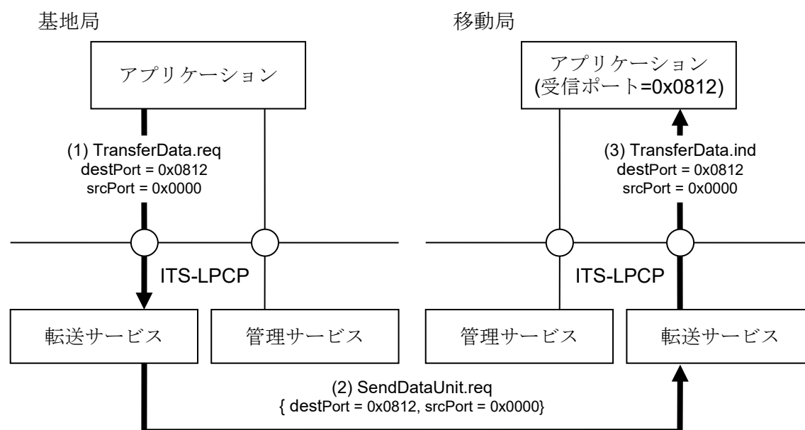
図 3.2-22 通信エリア進入
