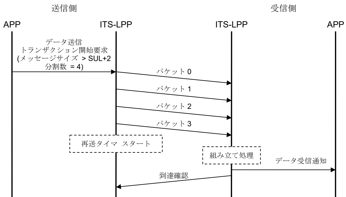
図 3.3-7 メッセージの分割・組立処理の例
