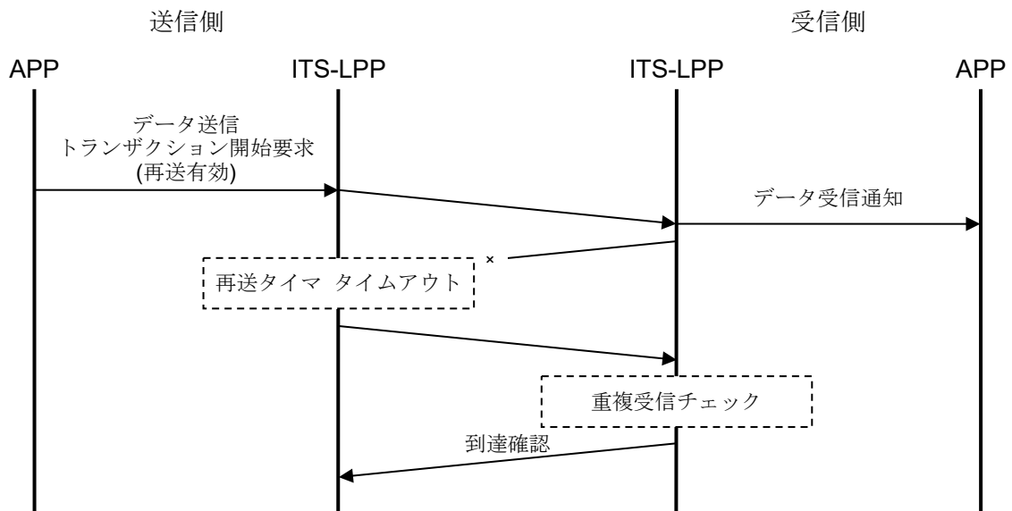
図 3.3-6 重複受信チェックの例
