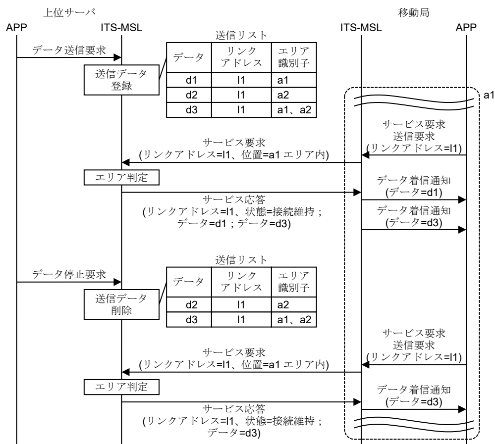
付図 D7-15 転送サービス処理手順の例（データの送信を停止）
