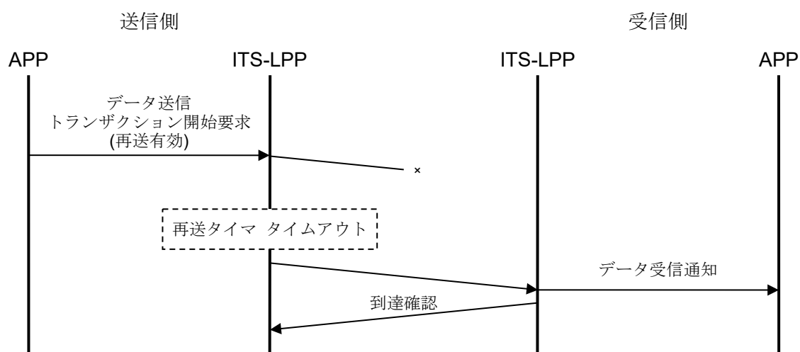
図 3.3-5 データ再送の例
