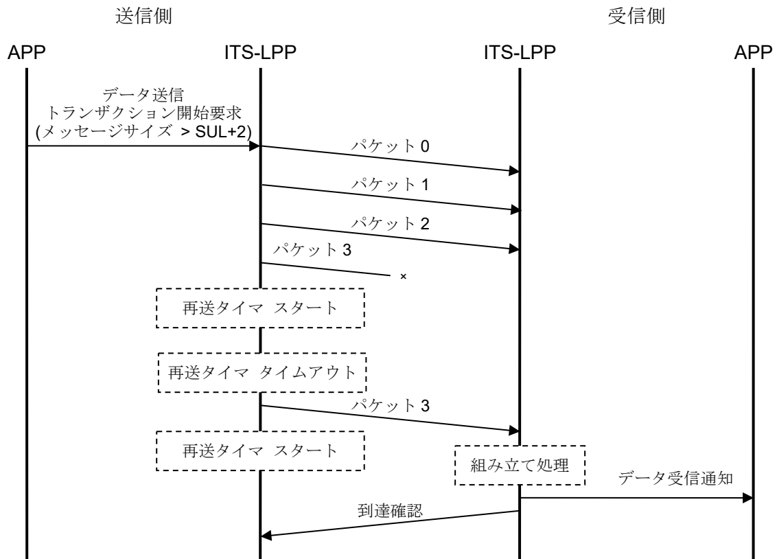
図 3.3-9 最終パケットの再送処理の例
