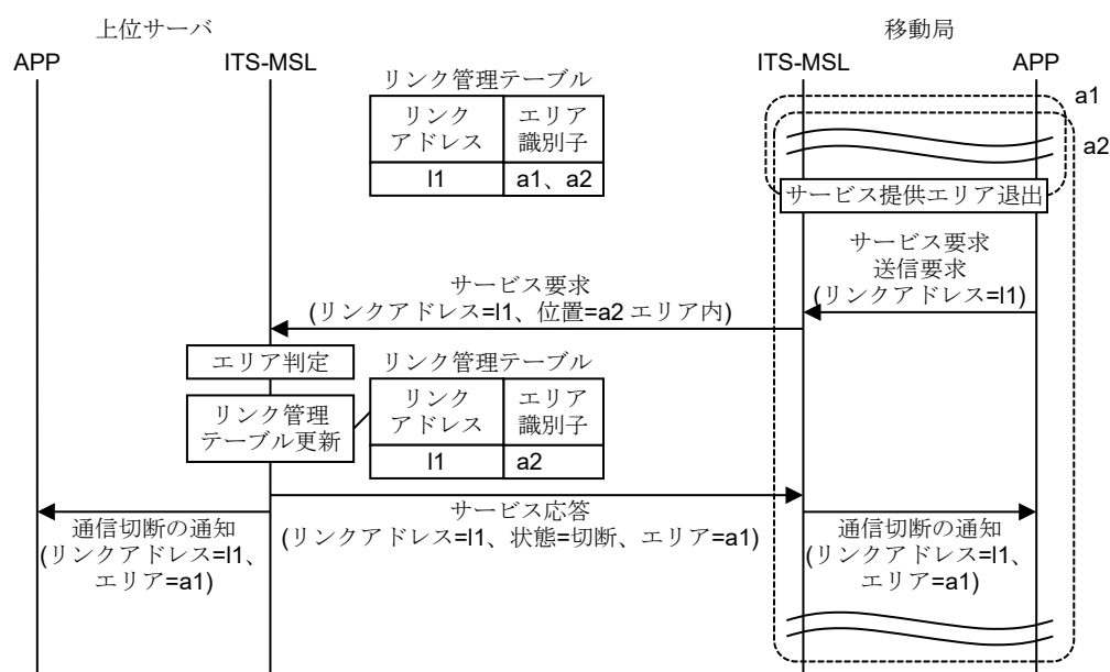
付図 D7-8 通信接続管理手順の例（サービス提供エリアから退出）
