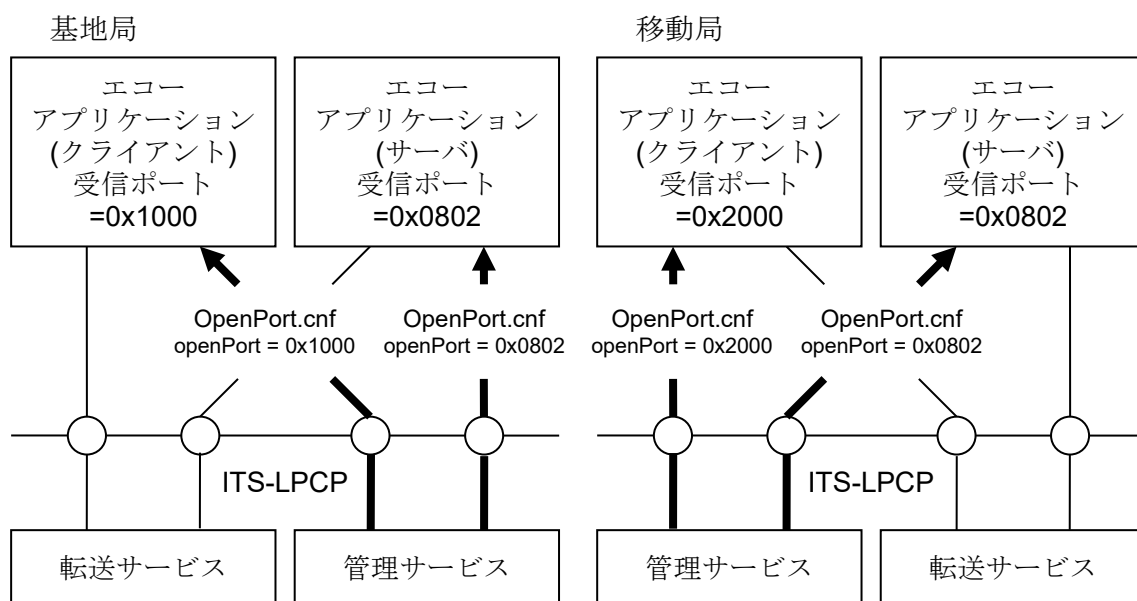
図 3.2-9 アプリケーション登録動作例 (その 2)
