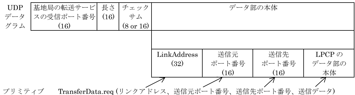
図 3.3-31 TransferDasta.req における PDU マッピング
