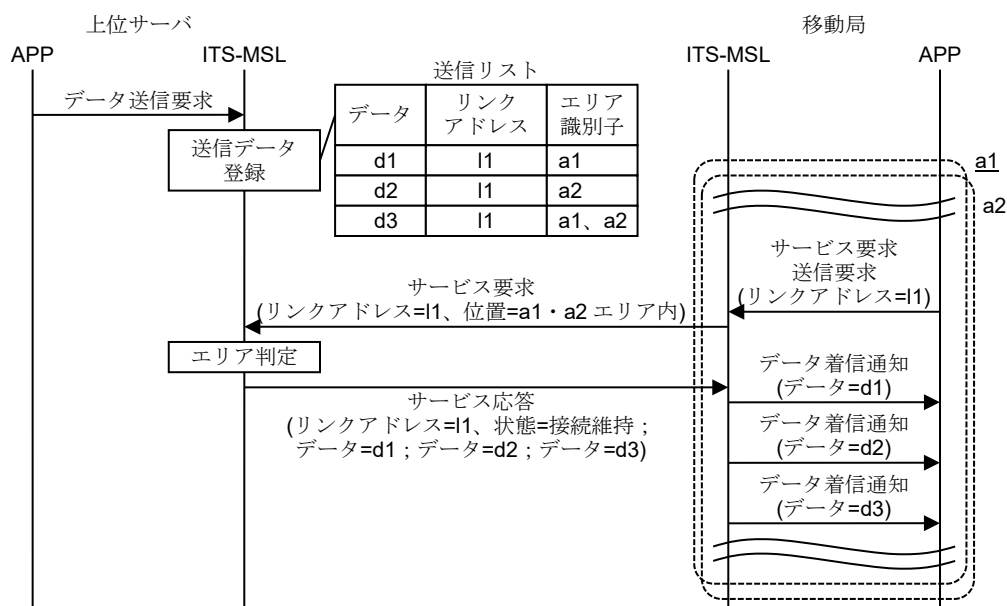
付図 D7-12 転送サービス処理手順の例 (重なったサービス提供エリア内を走行)
