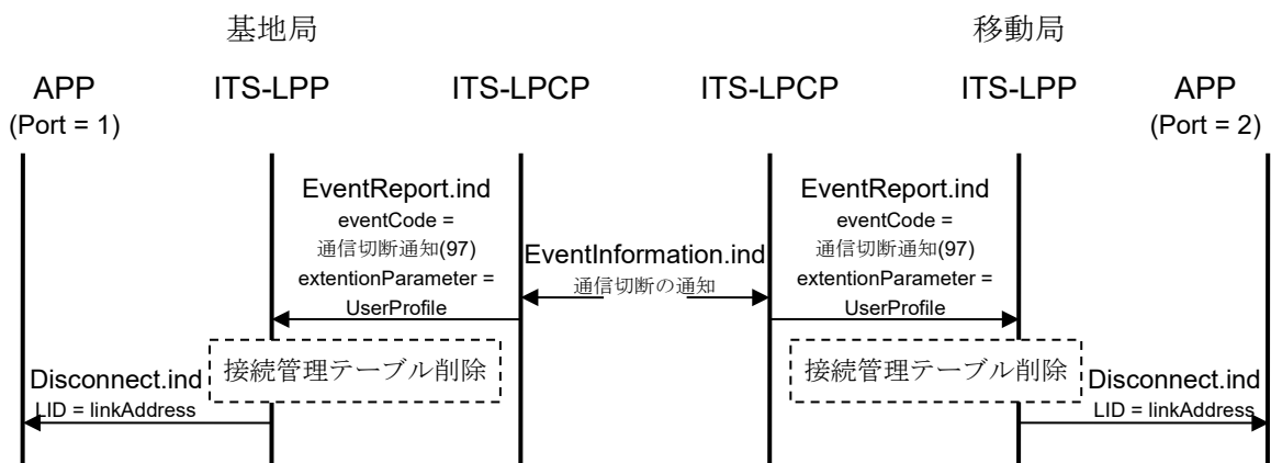
図 3.3-24 通信切断時の手順
