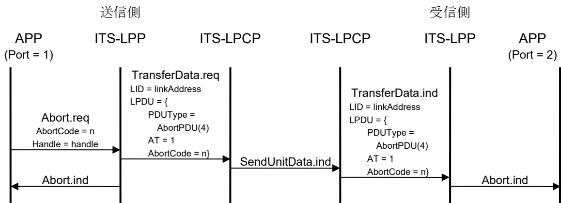
図 3.3-25 トランザクション破棄手順
