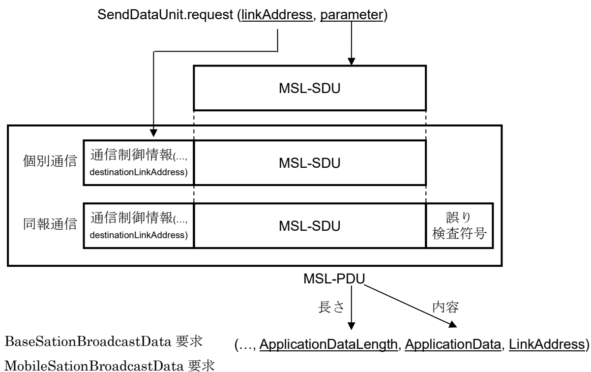
付図 F-1 SendDataUnit.request における下位層プリミティブへのマッピング
