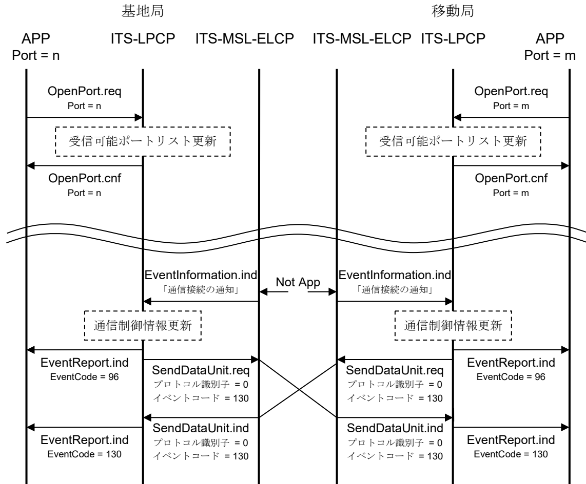
図 3.2-3 初期接続手順の概略
