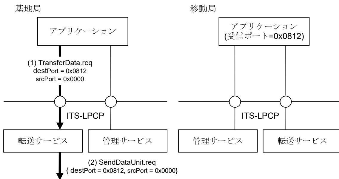
図 3.2-21 基地局側アプリケーションの起動
