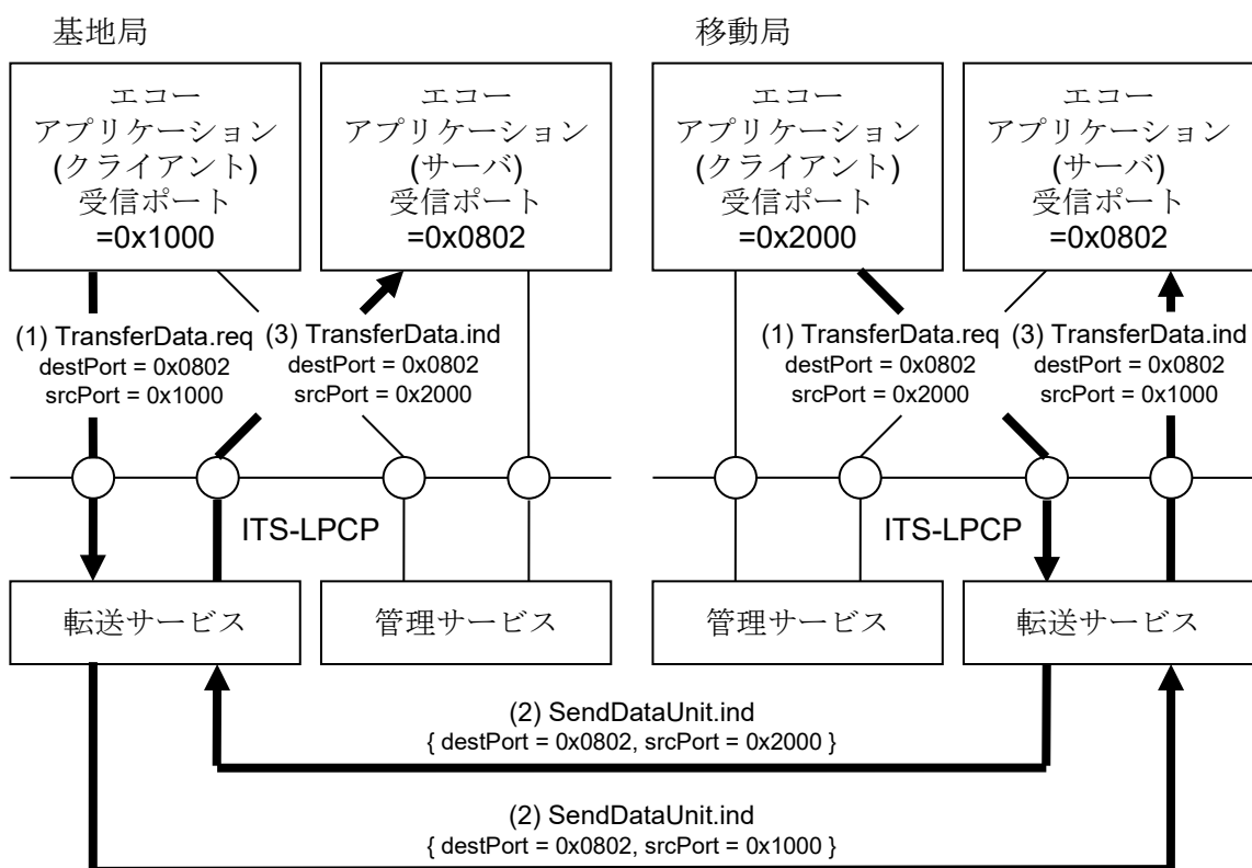
図 3.2-12 データ転送動作例 (エコー要求)
