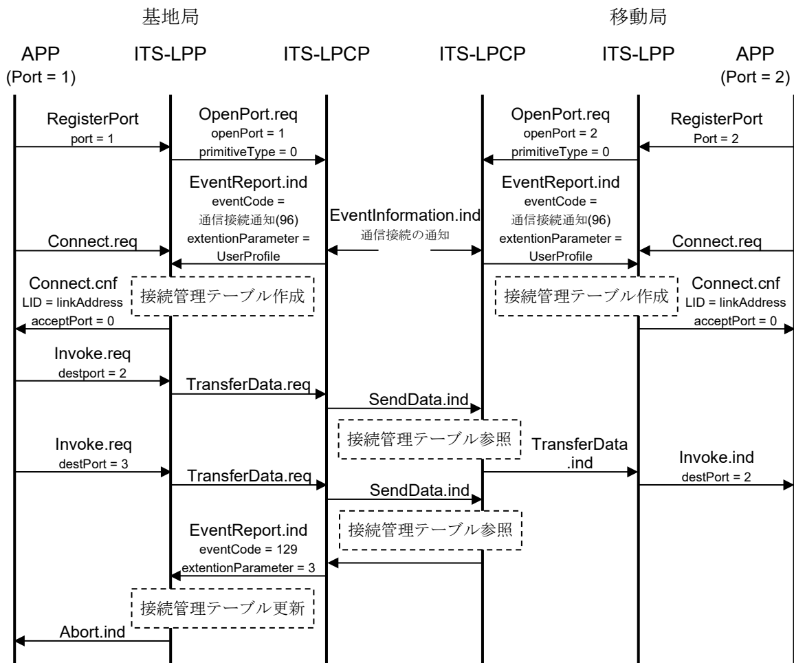
図 3.3-13 高速接続アプリケーションの初期接続シーケンス例
