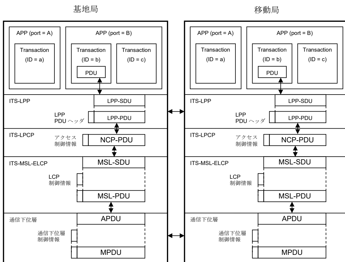
図 3.3-2 ITS-LPP におけるトランザクション間データ交換例
