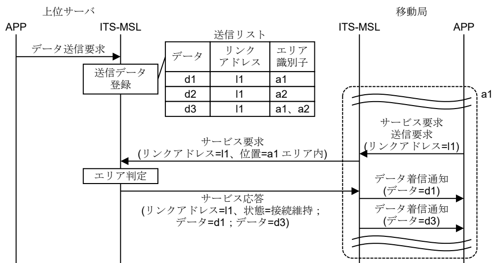
付図 D7-11 転送サービス処理手順の例 (単一のサービス提供エリア内を走行)
