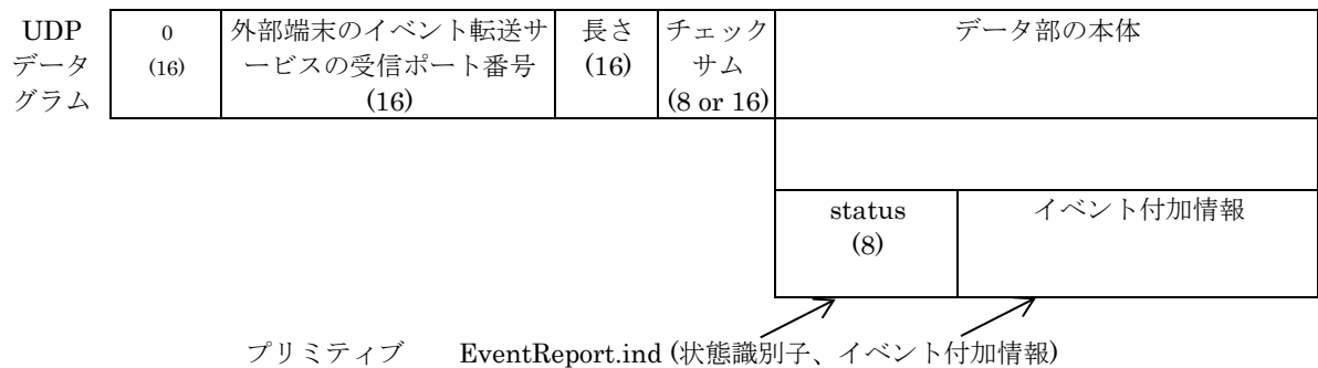
図 3.3-35 EventReport.ind における PDU マッピング
