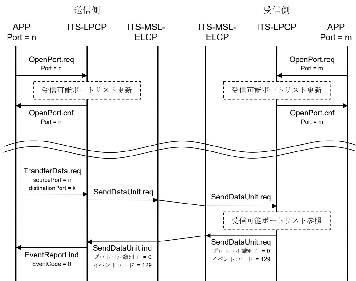
図 3.2-7 送信先ローカルポート番号が有効でない場合の処理手順の概略
