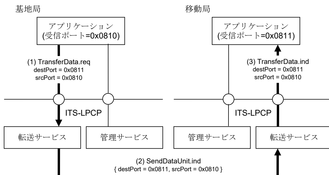
図 3.2-18 データ転送動作例 (基地局→移動局)
