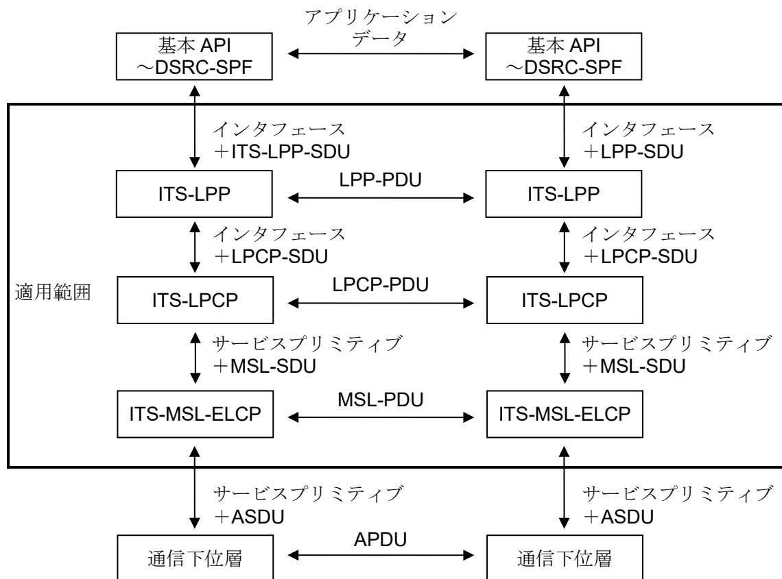
図 2.1-1 ITS-MSL のサービスインタフェースとプロトコルの概観
