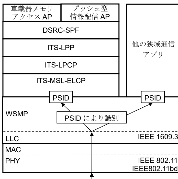
図 2.2-2 IEEE 802.11・IEEE802.11bd における伝送先アプリケーションの識別
