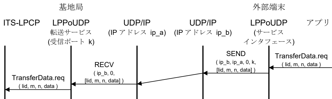
図 3.3-32 TransferData.req シーケンス
