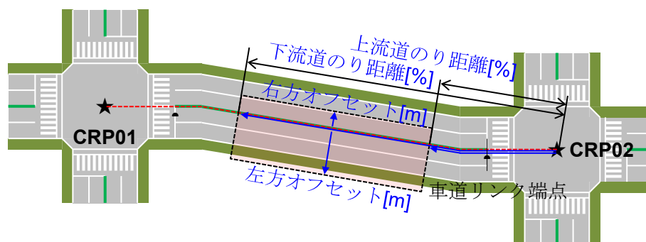
付図 D3-2 サービス提供エリアの位置表現イメージ (位置情報表現タイプ 2)
