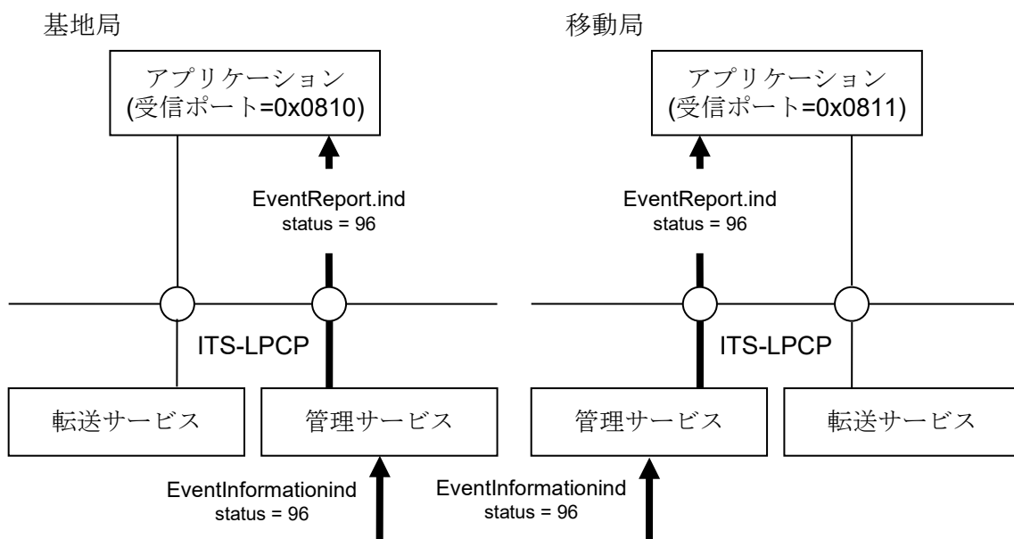
図 3.2-16 初期接続動作 (接続通知)
