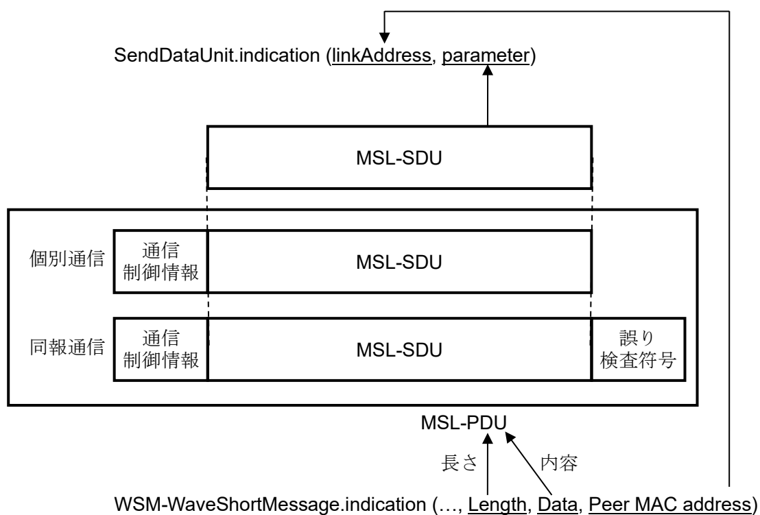
付図 C3-2 SendDataUnit.indication における下位層プリミティブへのマッピング
