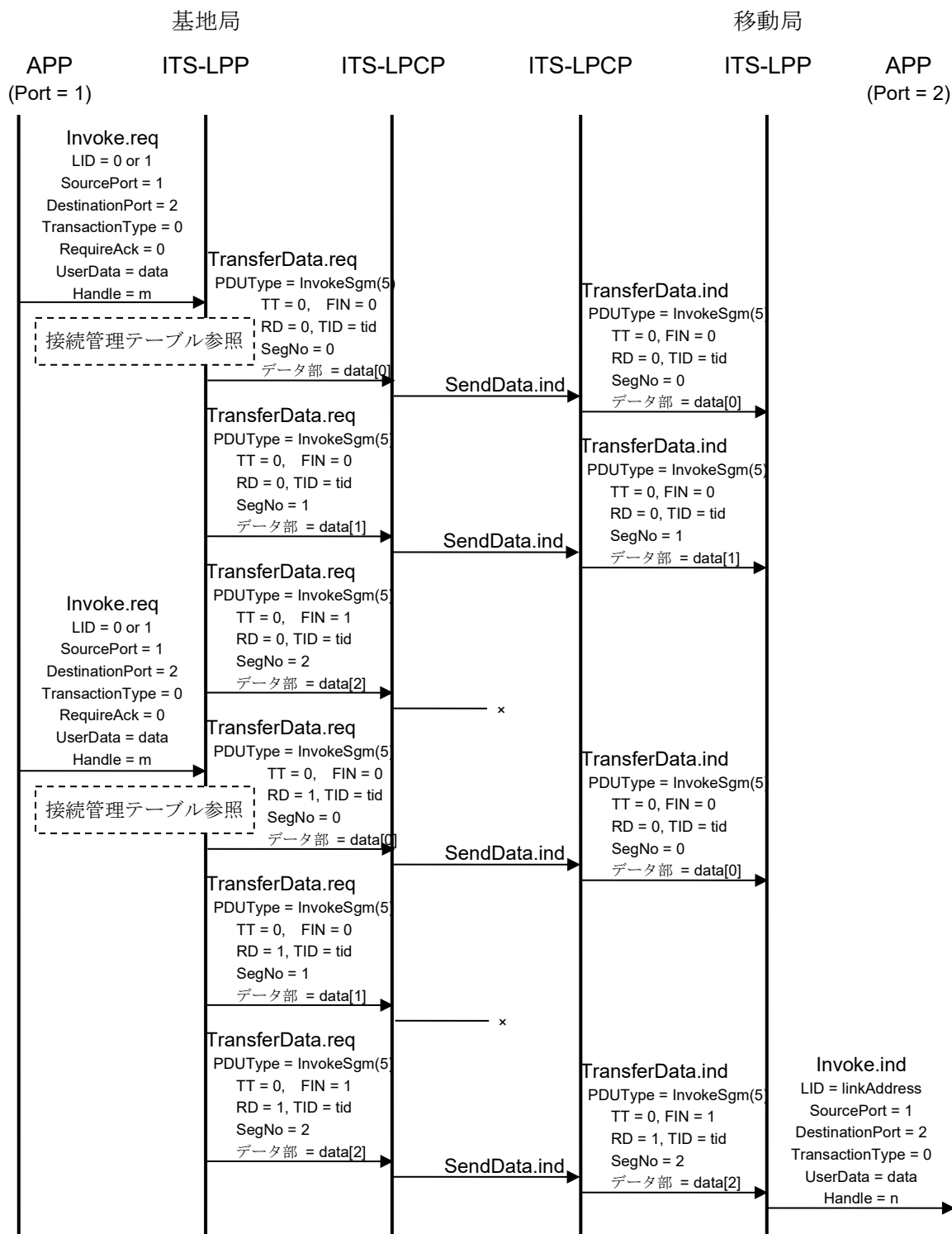
図 3.3-23 同報通信において分割・組立処理が有効な場合のシーケンス例
