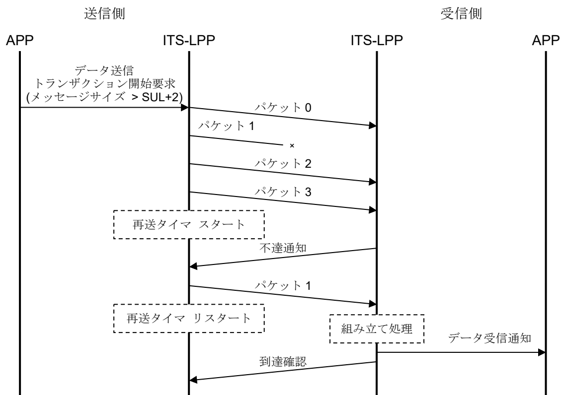
図 3.3-8 選択的再送処理の例
