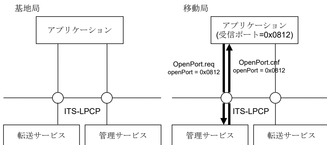
図 3.2-20 アプリケーション登録動作
