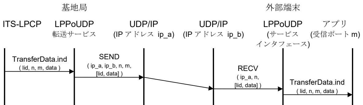
図 3.3-34 TransferData.ind シーケンス
