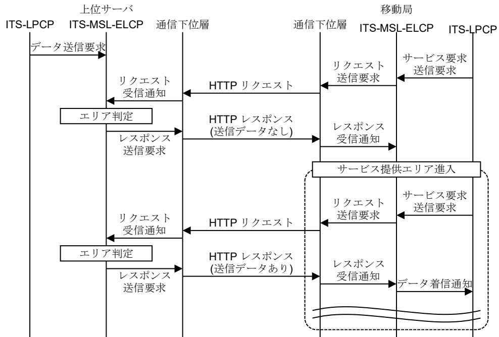
図 3.1-10 上位サーバから移動局への転送サービス処理手順の例
