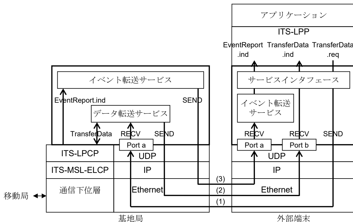
図 3.3-28 LPP over UDP の概要
