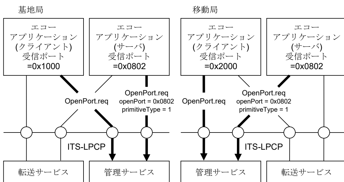
図 3.2-8 アプリケーション登録動作例（その 1）
