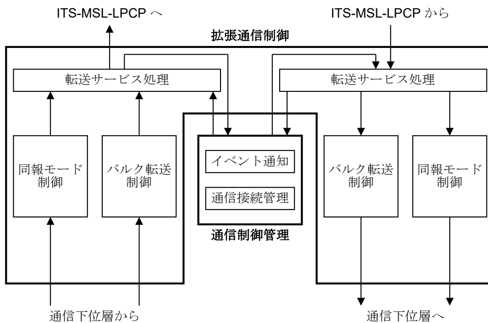
図 3.1-2 移動局における ITS-MSL-ELCP のエンティティ構成
