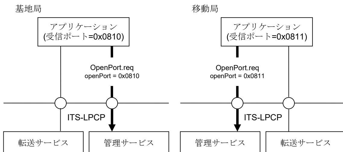
図 3.2-14 アプリケーション登録動作例 (その1)
