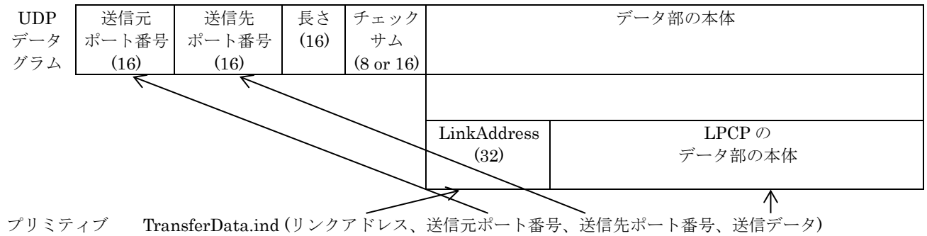
図 3.3-33 TransferData.ind における PDU マッピング
