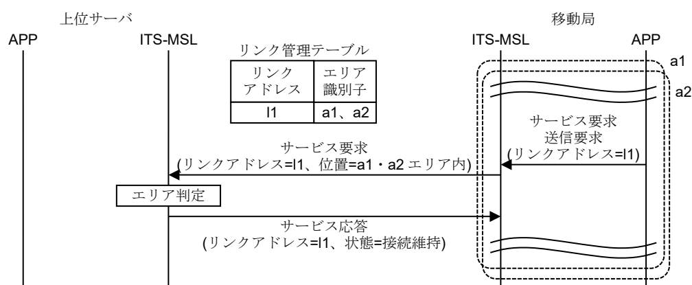
付図 D7-7 通信接続管理手順の例（サービス提供エリア内を走行）
