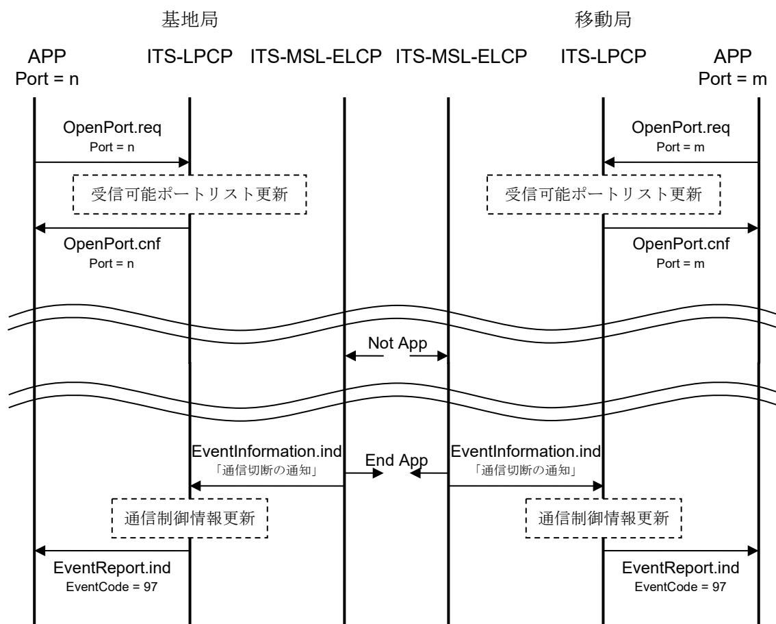
図 3.2-4 通信終了手順の概略
