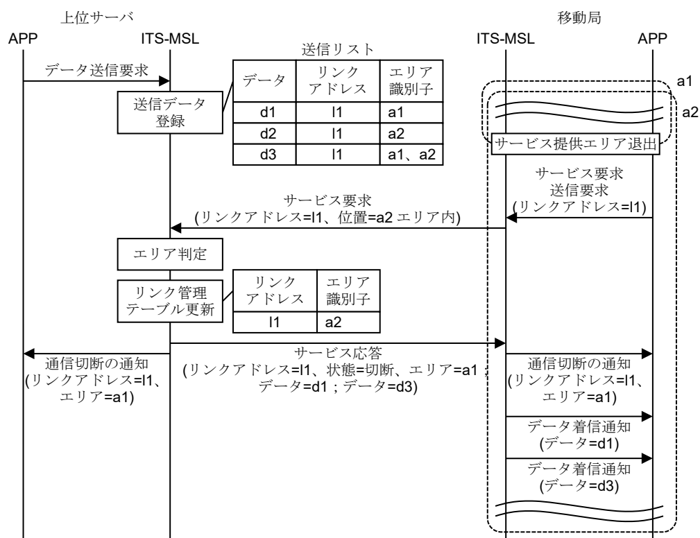
付図 D7-14 転送サービス処理手順の例（サービス提供エリアから退出）
