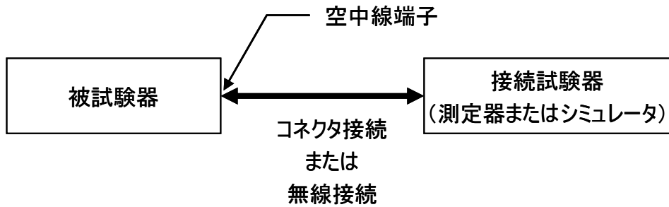
図 2-2 通信制御方式に関する試験構成
