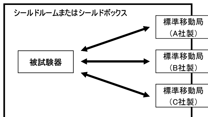
図 4-1 無線接続で Interoperability 試験を実施する試験構成例
