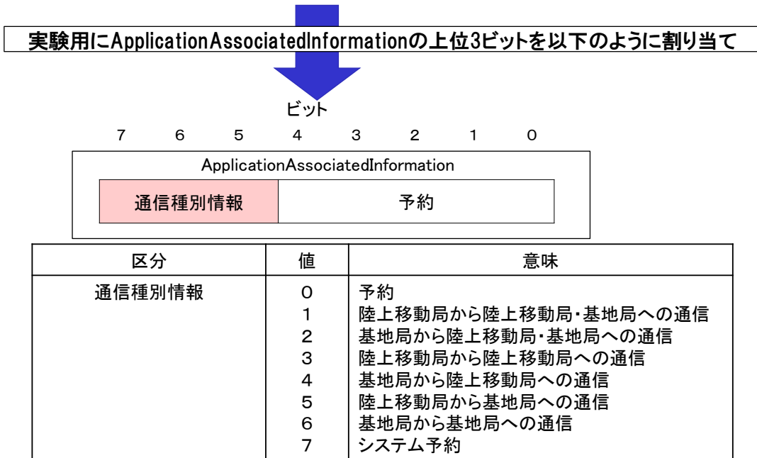
図4-29 ApplicationAssociatedInformation の構成
