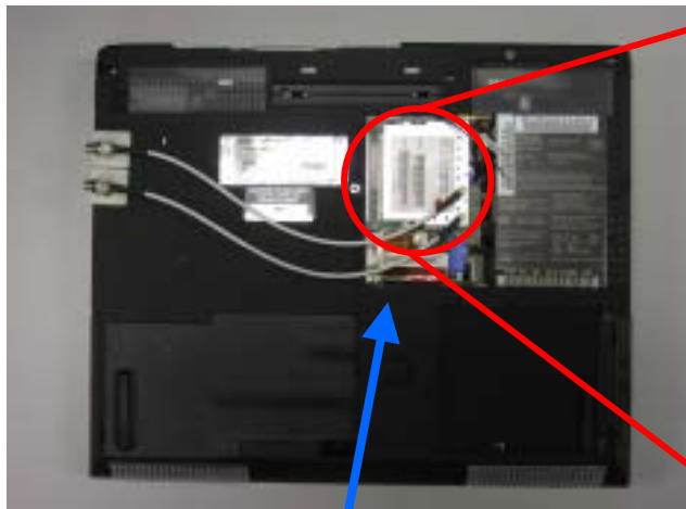
MiniPCI format 802.11a card
